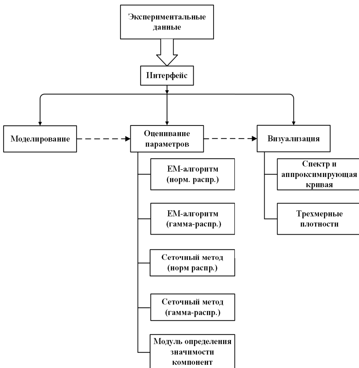
Рис. 7.16. Структура информационной технологии
