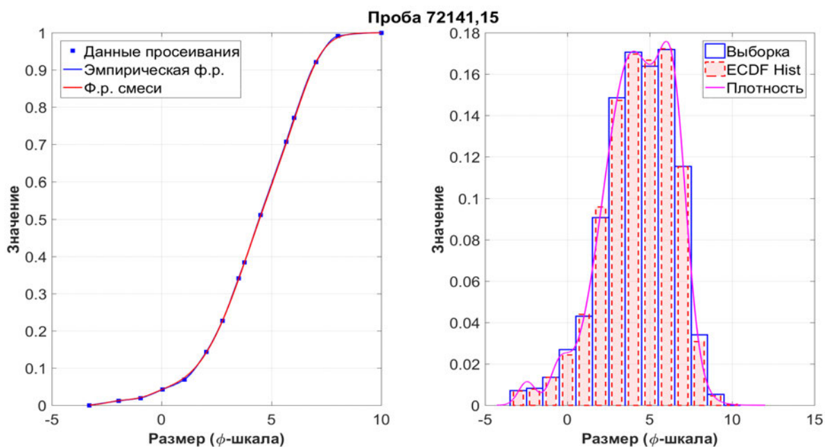
Рис. 4.8. Проба лунного грунта 72141,15 (миссия «Аполлон-17»)
