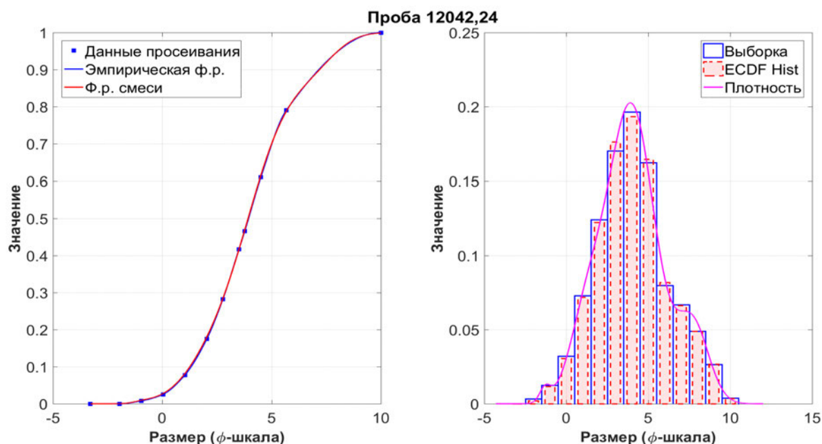
Рис. 4.1. Проба лунного грунта 12042,24 (миссия «Аполлон-12»)
