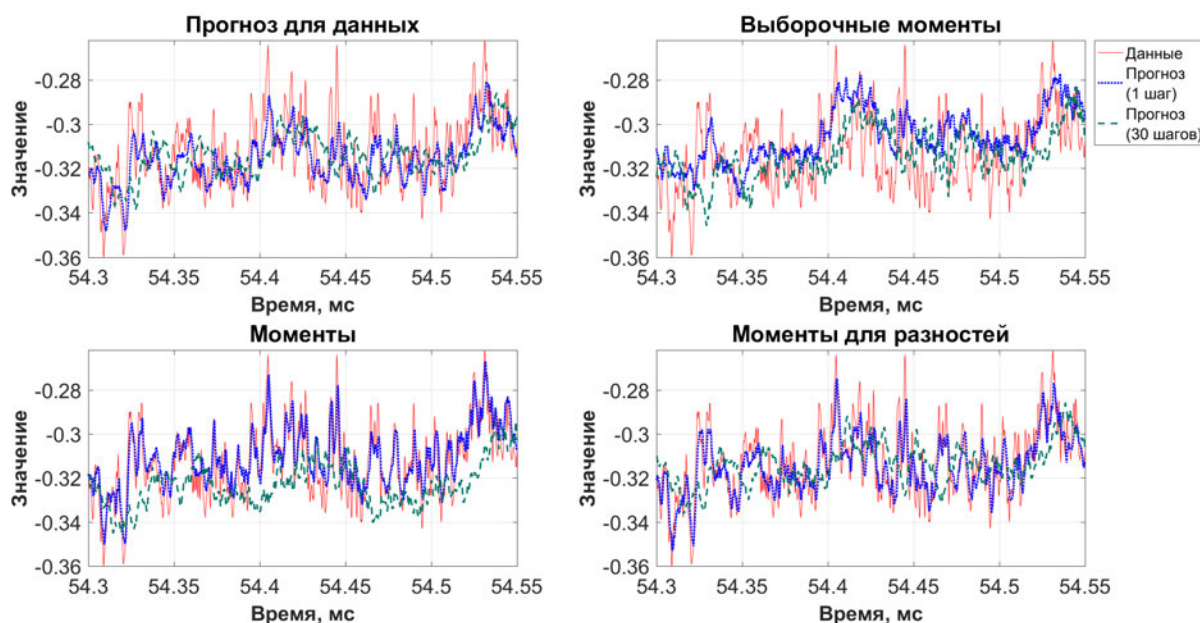
Рис. 5.21. Пример прогноза для ряда A19692 (54,30–54,55 мс)
