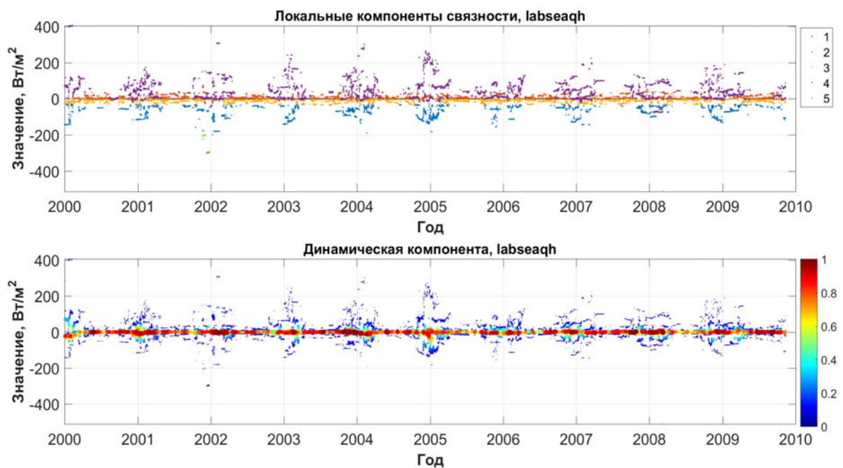
Рис. 6.59. Оценки распределения сдвига (Лабрадорское море, скрытые потоки)
