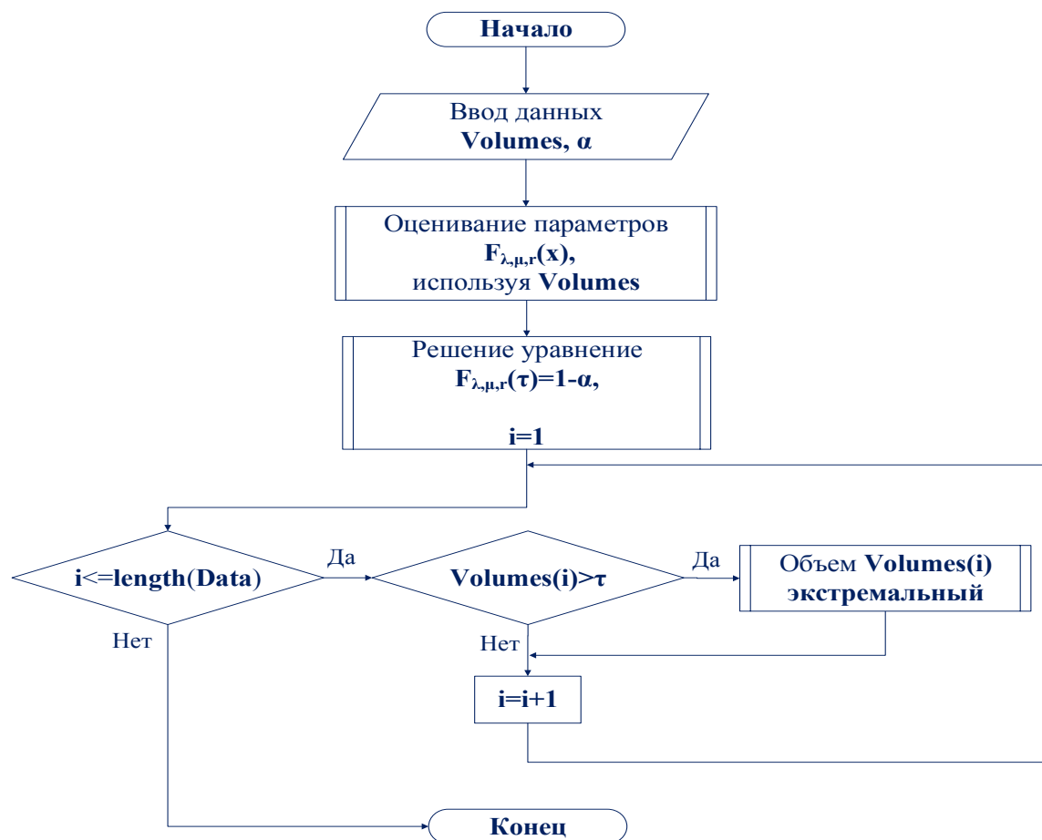
Рис. 6.46. Процедура определения аномальности объемов осадков
