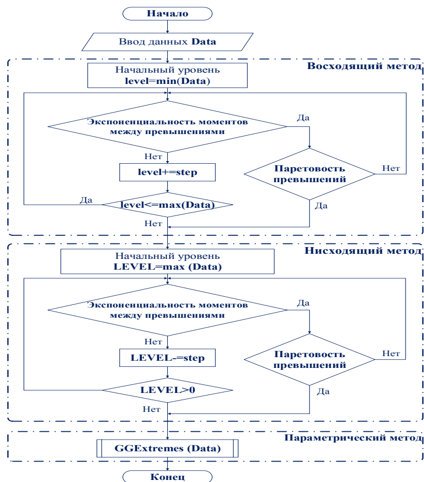
Рис. 6.32. Процедура идентификации экстремальных наблюдений
