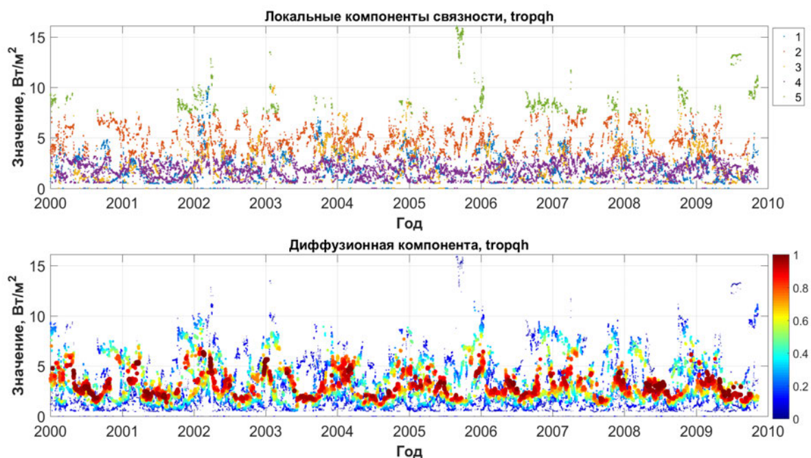
Рис. 6.64. Оценки распределения коэффициента диффузии (тропики, явные потоки)
