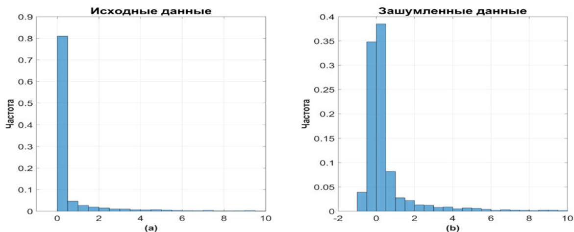
Рис. 3.11. Гистограммы для исходных и зашумленных данных
