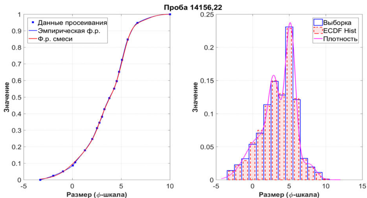
Рис. 4.2. Проба лунного грунта 14156,22 (миссия «Аполлон-14»)
