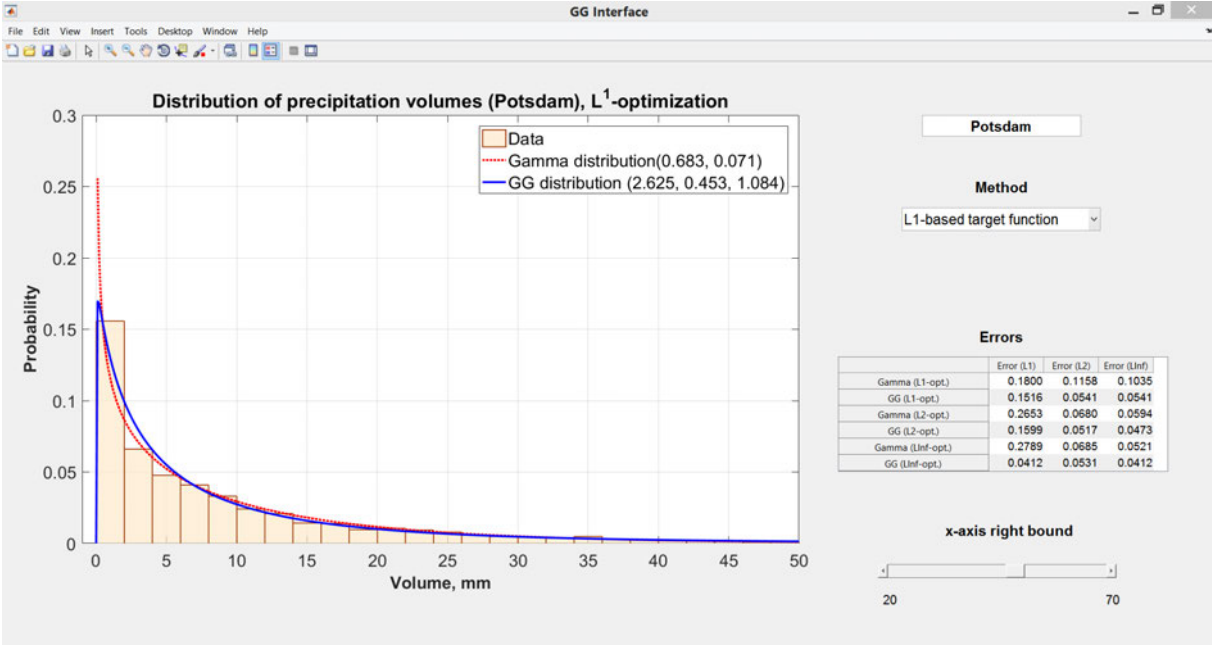
Рис. 7.13. Аппроксимация распределения объемов осадков за дождливые периоды на основе метрики L^1
