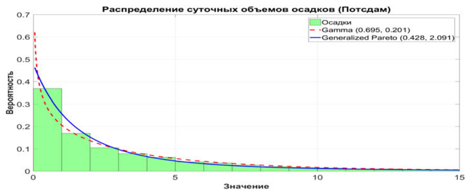
Рис. 6.20. Распределение суточных объемов осадков, Потсдам
