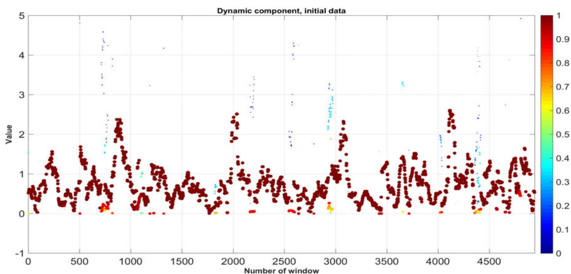
Рис. 3.12. Динамическая компонента, исходные данные
