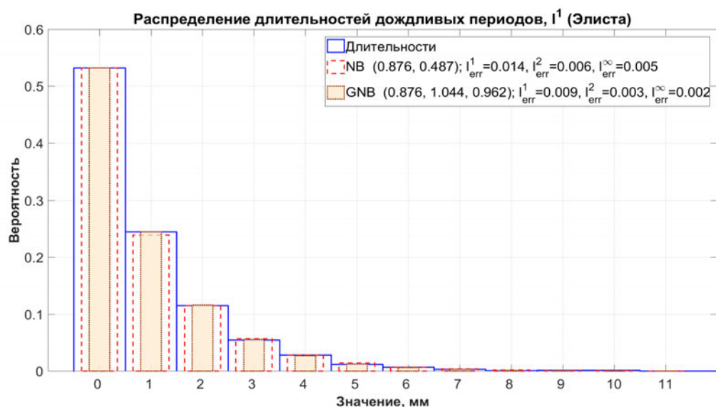
Рис. 6.25. Распределение длительностей «дождливых» периодов в Элисте, пример аппроксимации в \ell^1
