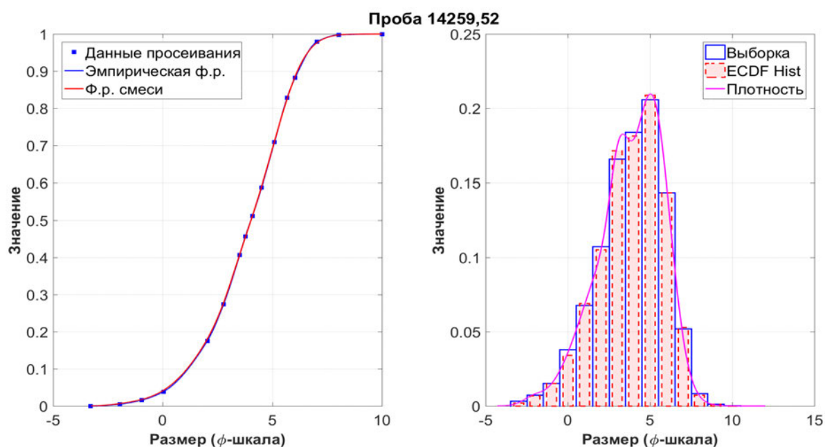
Рис. 4.3. Проба лунного грунта 14259,52 (миссия «Аполлон-14»)
