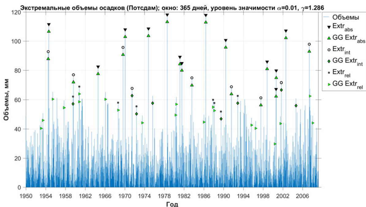
Рис. 6.37. Аномальные объемы осадков, окно 365 дней (Потсдам)
