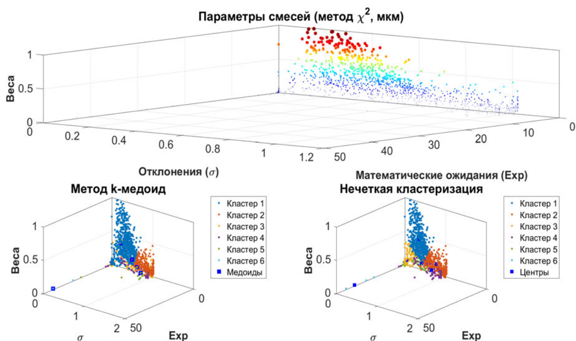
Рис. 4.28. Кластеризация параметров в пространстве (метод \chi^2 , мкм) определенное сходство прослеживается для достаточно большого числа столбцов, при этом наиболее близкие значения получены при кластеризации параметров в микрометрах при аппроксимации на основе статистики \chi^2 (см. правый столбец в таблице 4.2). Результаты нечеткой кластери-
