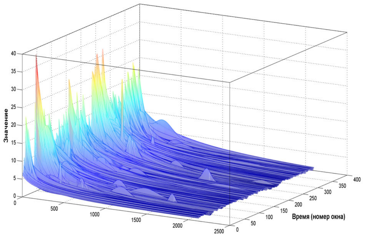
Рис. 2.1. Эволюция плотности смеси гамма-распределений
