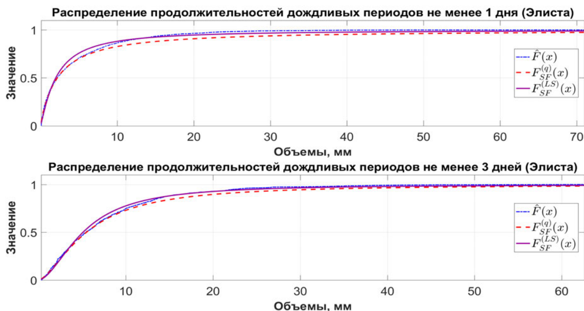
Рис. 6.45. Аппроксимация асимптотическим распределением, Элиста
