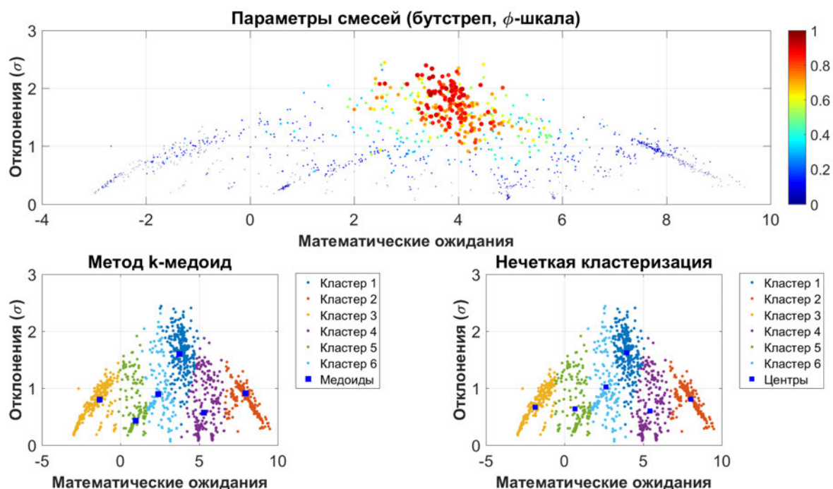
Рис. 4.21. Кластеризация параметров смесей (бутстреп, \phi -шкала)
