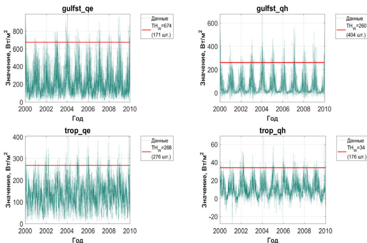
Рис. 6.67. Пороговые значения для потоков тепла
