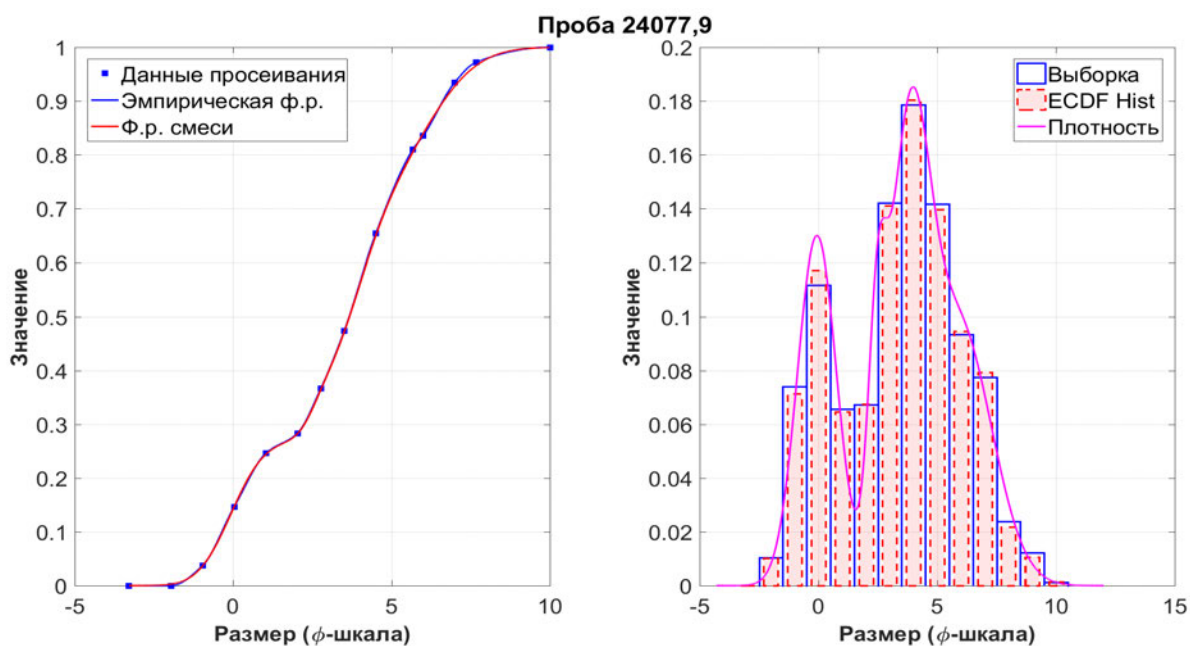
Рис. 4.6. Проба лунного грунта 24077,9 (миссия «Луна-24»)
