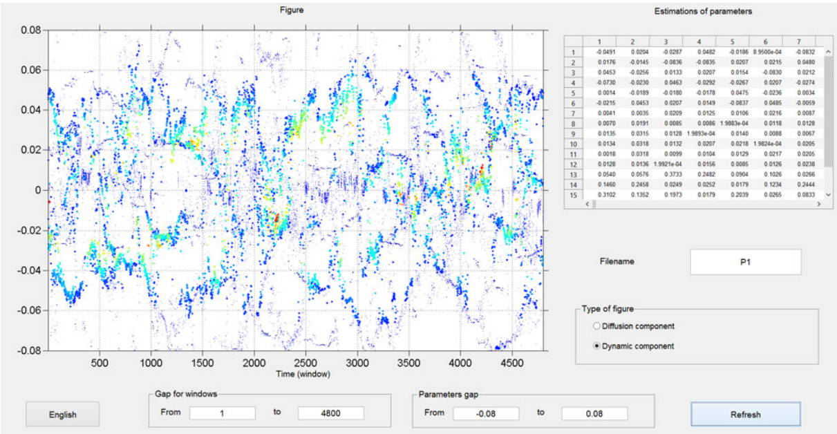
Рис. 7.7. Пример: динамическая компоненты
