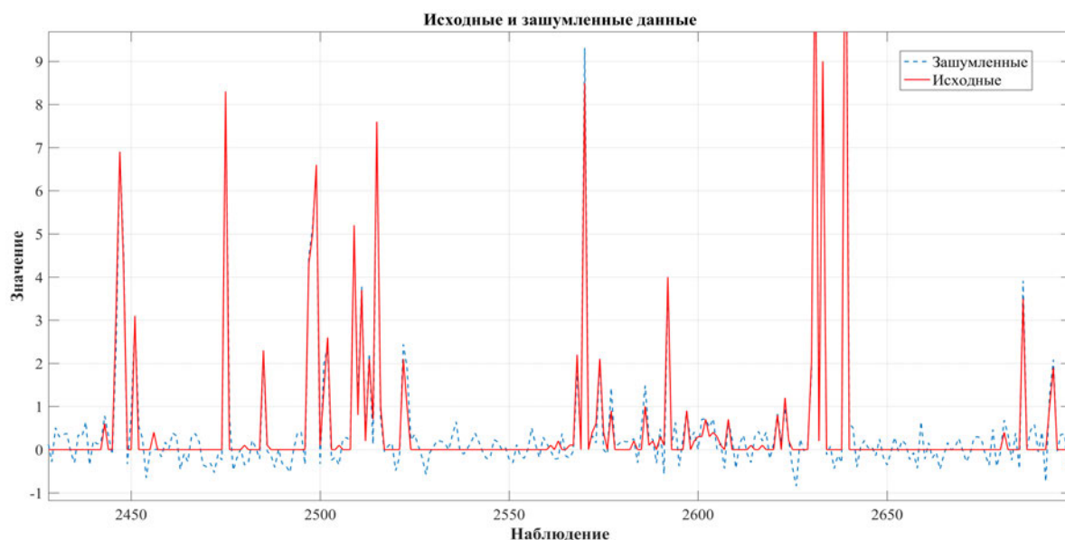
Рис. 3.10. Исходные и зашумленные данные для объемов осадков
