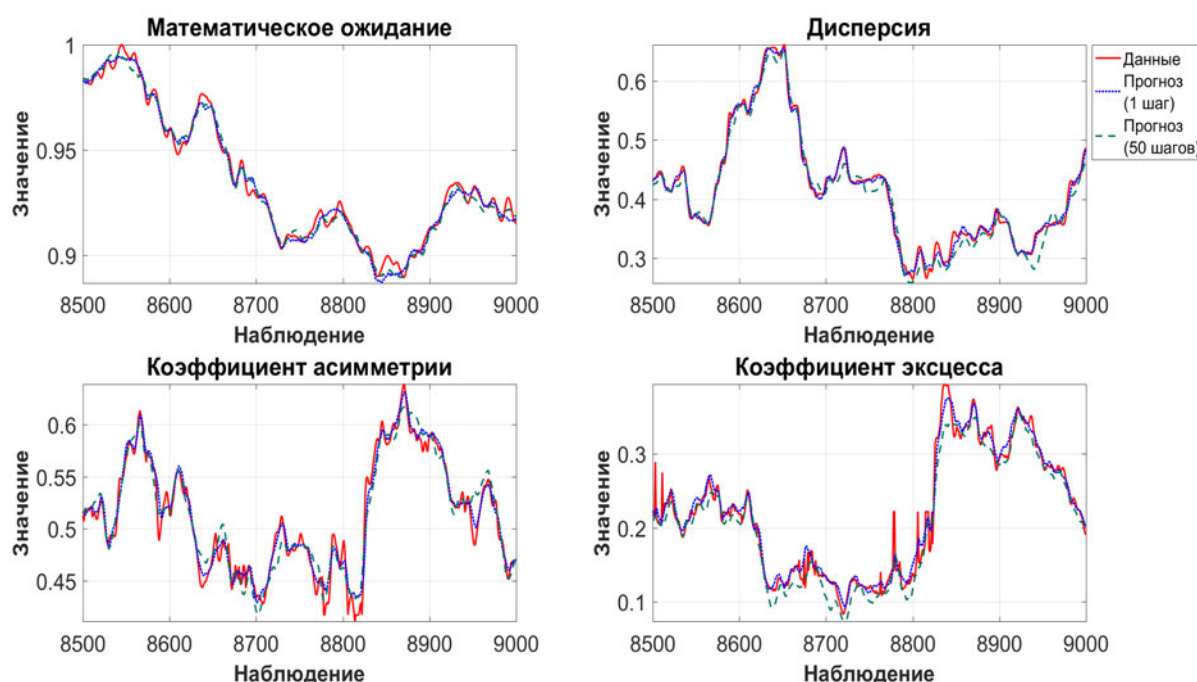
Рис. 5.29. Сравнение значений исходных данных (1), прогноза на 1 шаг (2) и на 50 шагов (3) для четырех моментов
