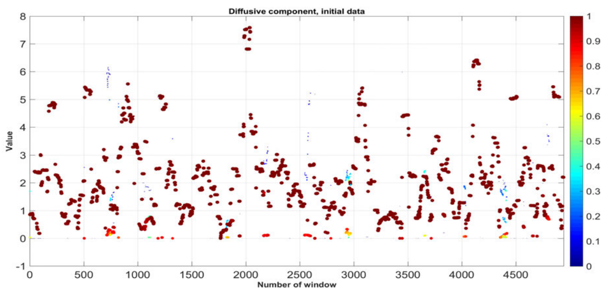
Рис. 3.13. Диффузионная компонента, исходные данные
