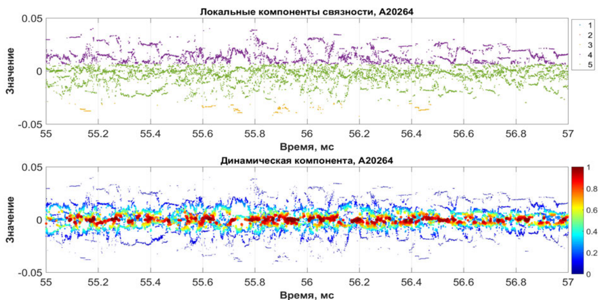
Рис. 5.14. Ансамбль A20264, динамическая компонента (55–57 мс)
