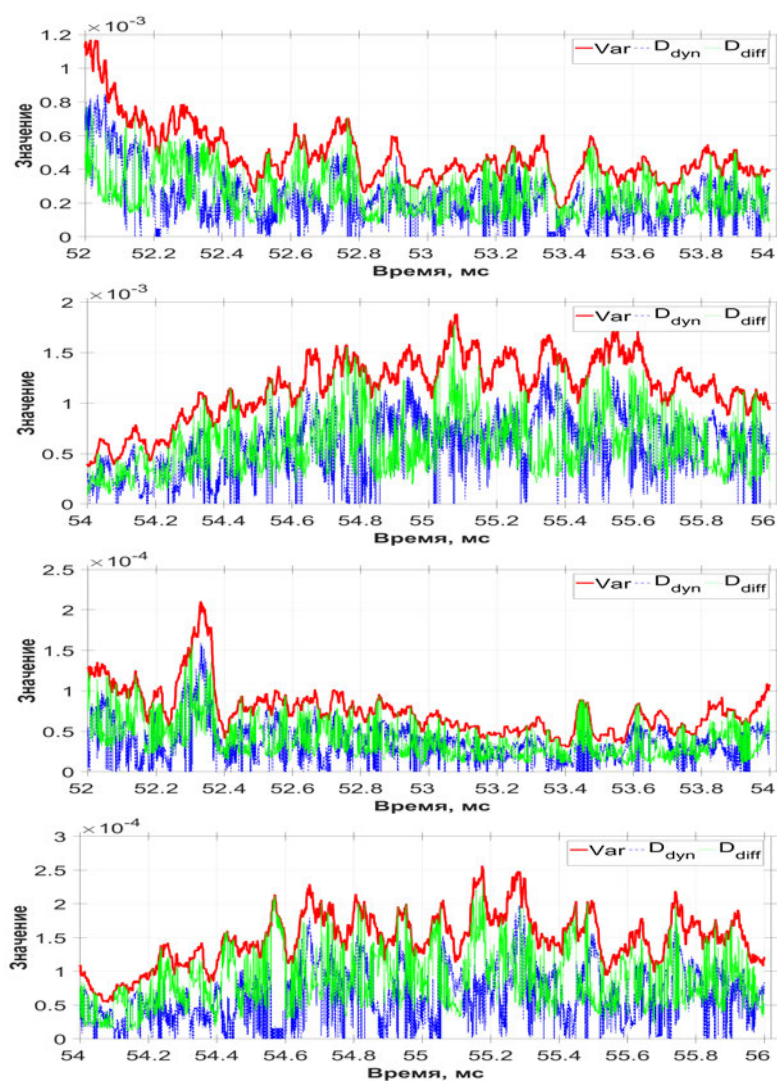
Рис. 5.19. Динамическая и диффузионная компоненты для двух областей
