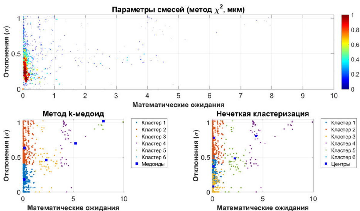
Рис. 4.24. Кластеризация параметров смесей (метод \chi^2 , мкм)
