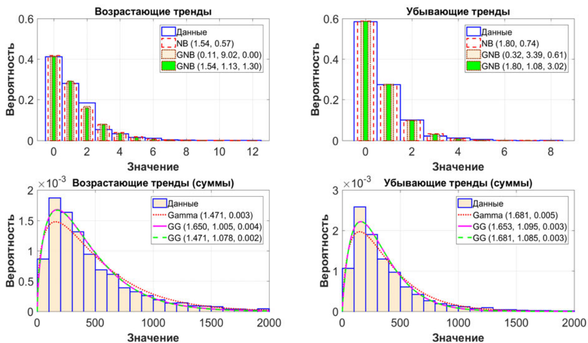
Рис. 6.71. Распределения характеристик (тропики, скрытые потоки)
