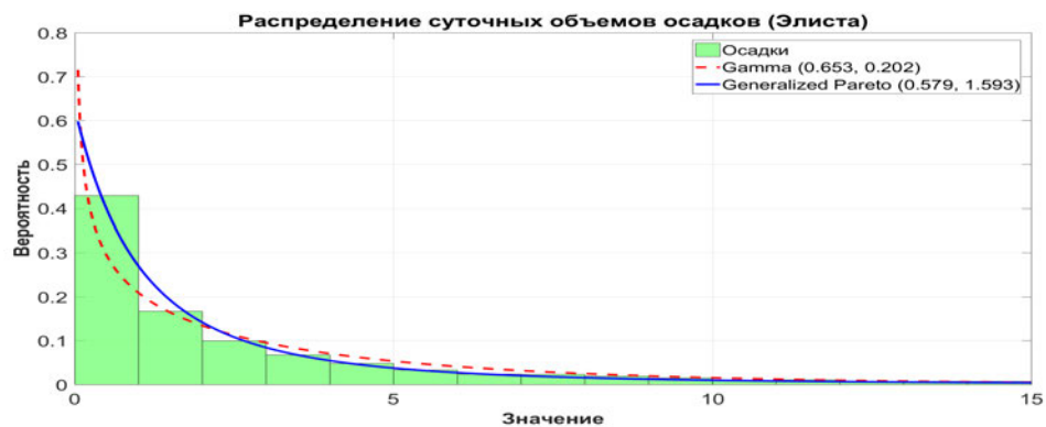
Рис. 6.21. Распределение суточных объемов осадков, Элиста
