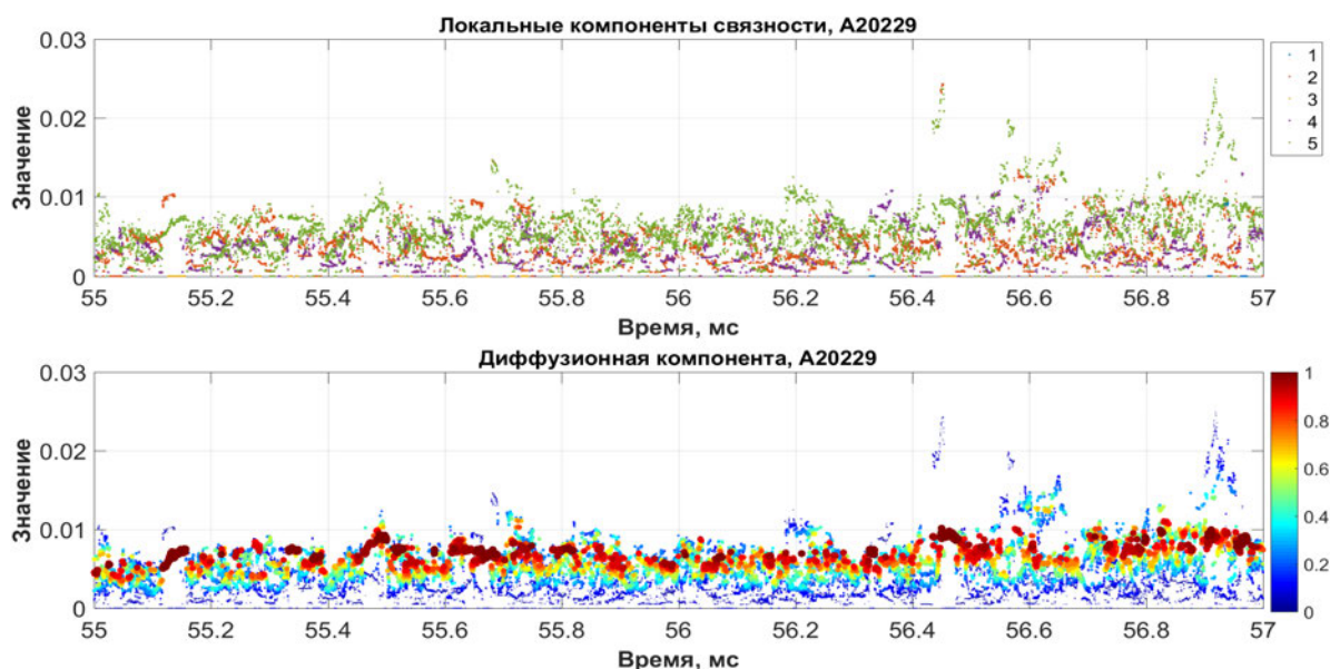
Рис. 5.11. Ансамбль A20229, диффузионная компонента (55–57 мс)
