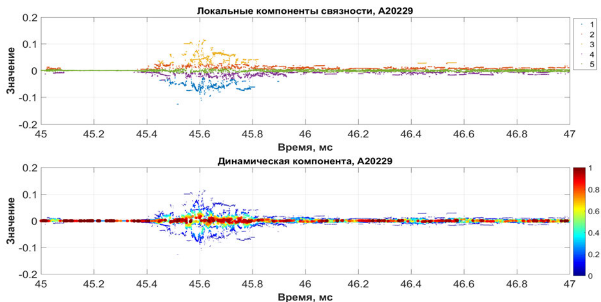
Рис. 5.8. Ансамбль A20229, динамическая компонента (45–47 мс)
