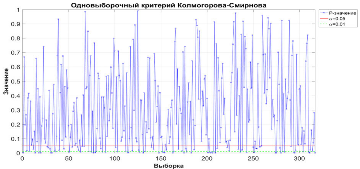
Рис. 4.10. Ошибки аппроксимации (критерий Колмогорова)
