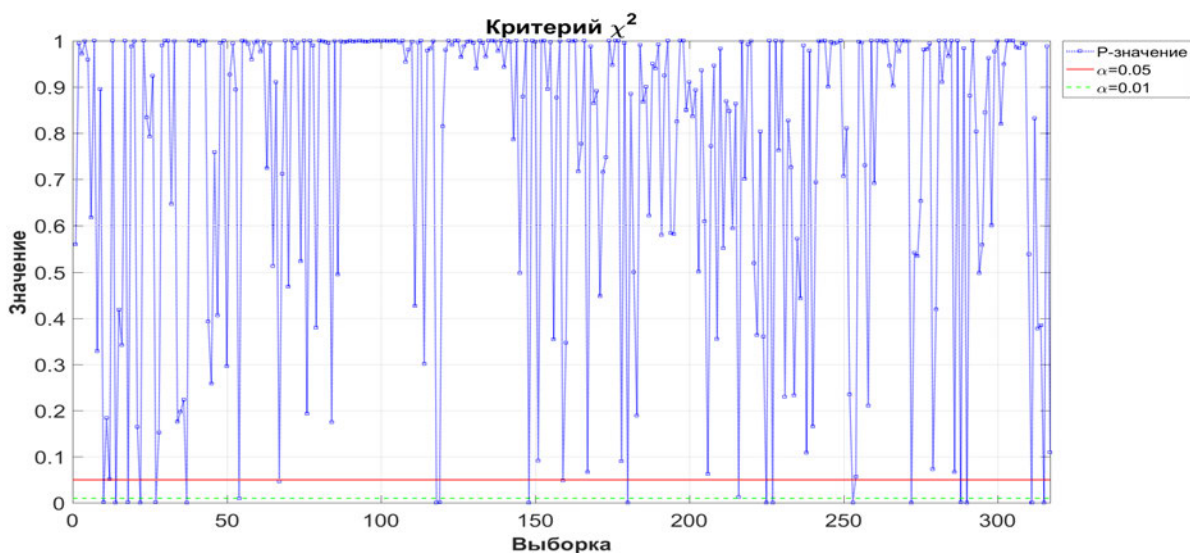
Рис. 4.20. Ошибки аппроксимации (критерий \chi^2 )
