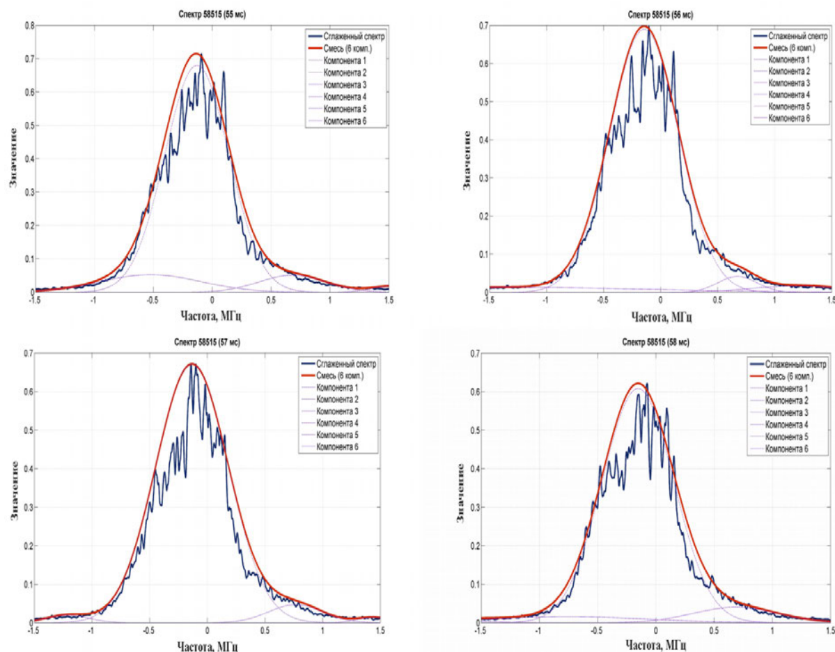
Рис. 5.1. Аппроксимация спектра 58515 с 55 мс по 58 мс
