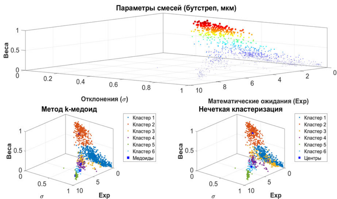
Рис. 4.27. Кластеризация параметров в пространстве (бутстреп, мкм)
