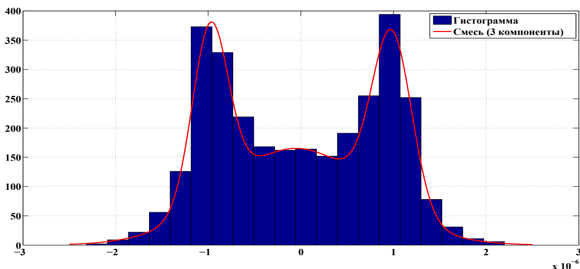
Рис. 3.6. Гистограмма для динамической компоненты волатильности для этапа до начала эксперимента с аппроксимирующей трехкомпонентной нормальной смесью
