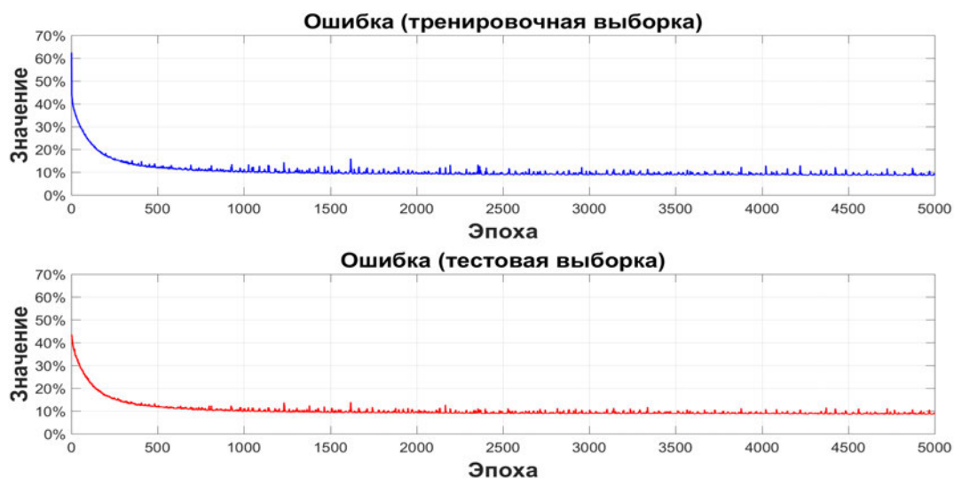
Рис. 6.6. Ошибки для однодневного прогноза, Потсдам
