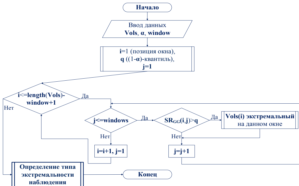
Рис. 6.32. Процедура идентификации экстремальных наблюдений
