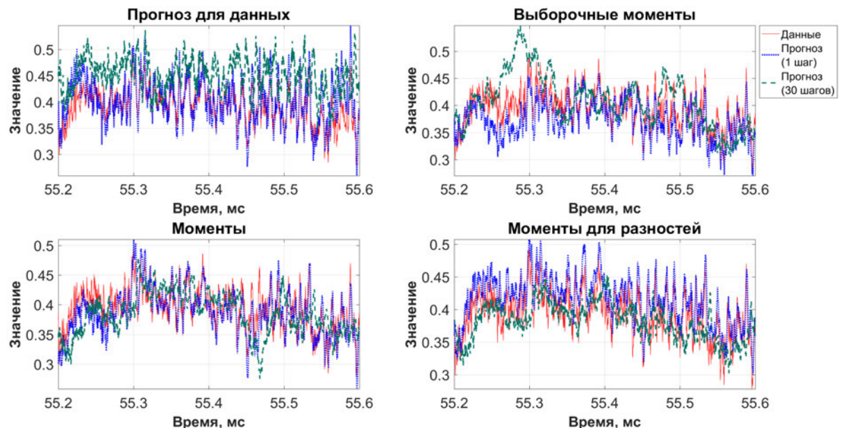
Рис. 5.23. Пример прогноза для ряда A20264 (55,20–55,60 мс)
