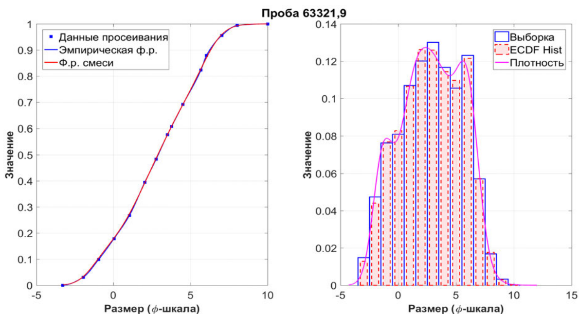
Рис. 4.7. Проба лунного грунта 63321,9 (миссия «Апполон-16»)
