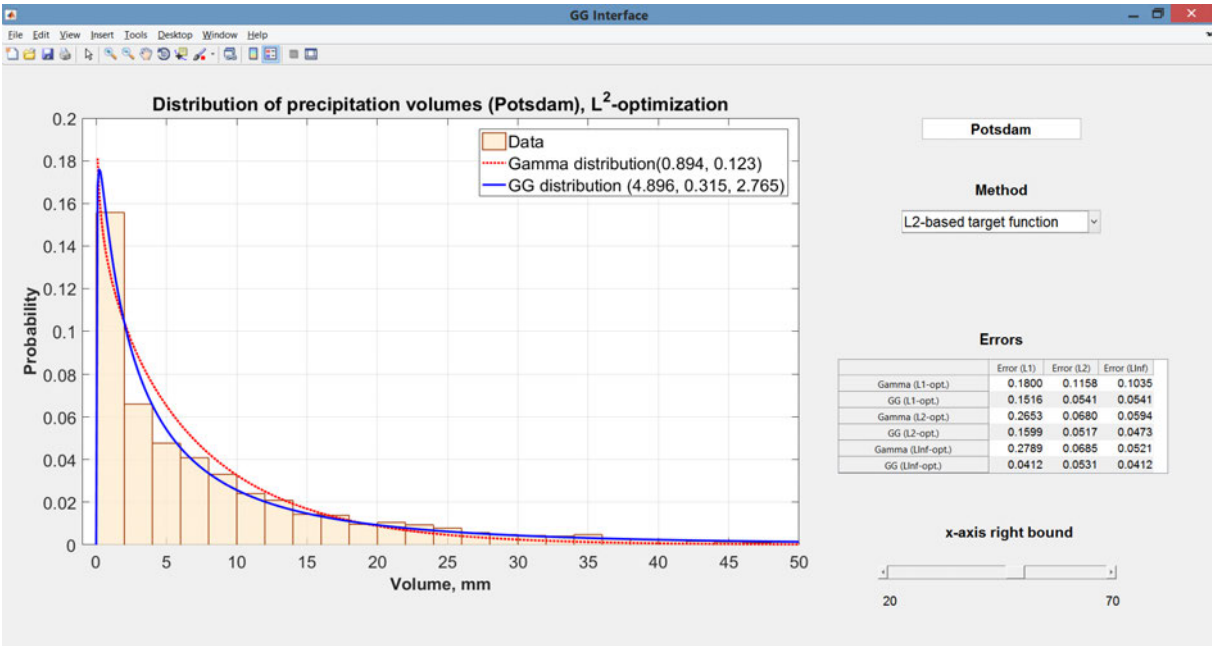
Рис. 7.14. Аппроксимация распределения объемов осадков за дождливые периоды на основе метрики L^2
