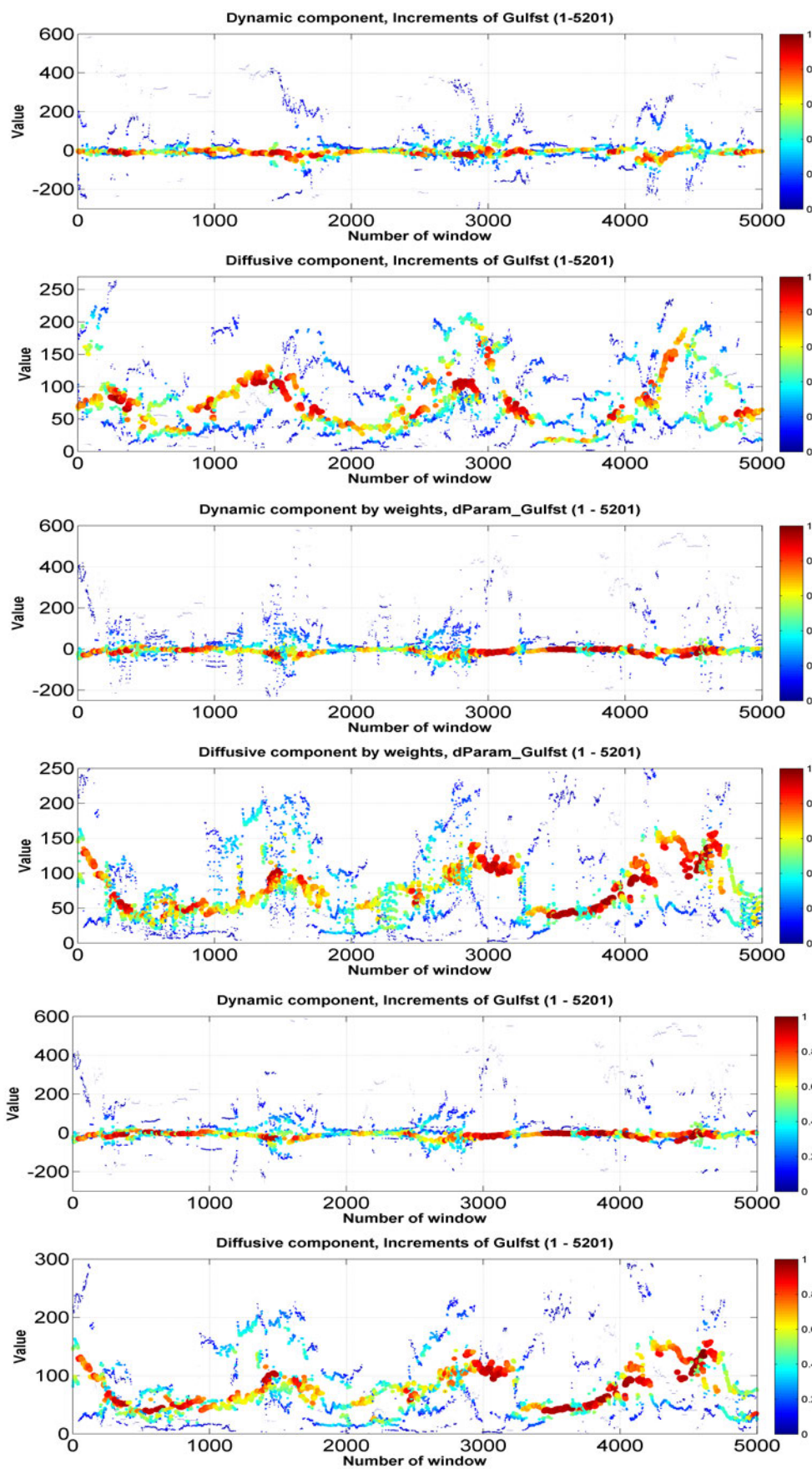
Рис. 6.51. СРС-оценки, полученные тремя модификациями классического ЕМ-алгоритма
