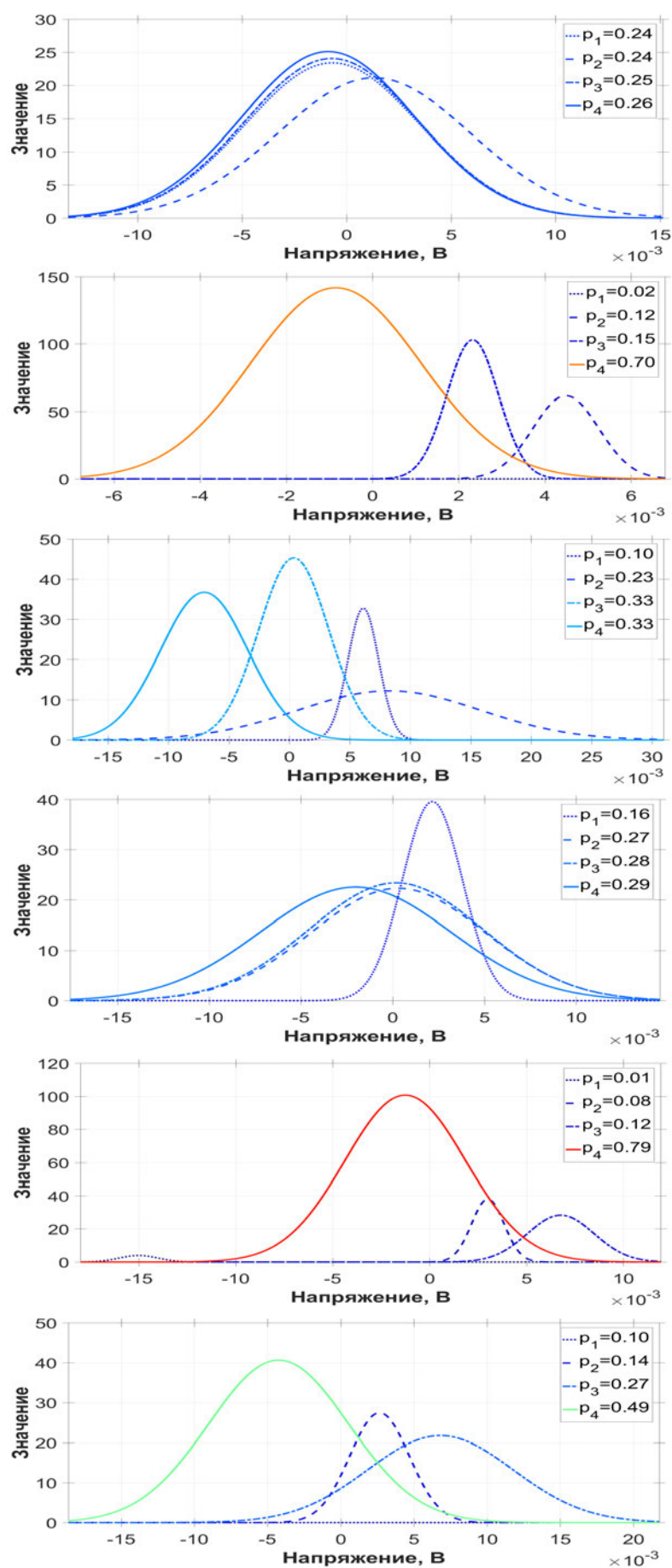
Рис. 5.17. Плотности для временных интервалов 52,00–52,04 мс, 53,8–53,84 мс, 54,42–54,46 мс, 54,5–54,54 мс, 57,8–57,84 мс и 57,94–58,98 мс
