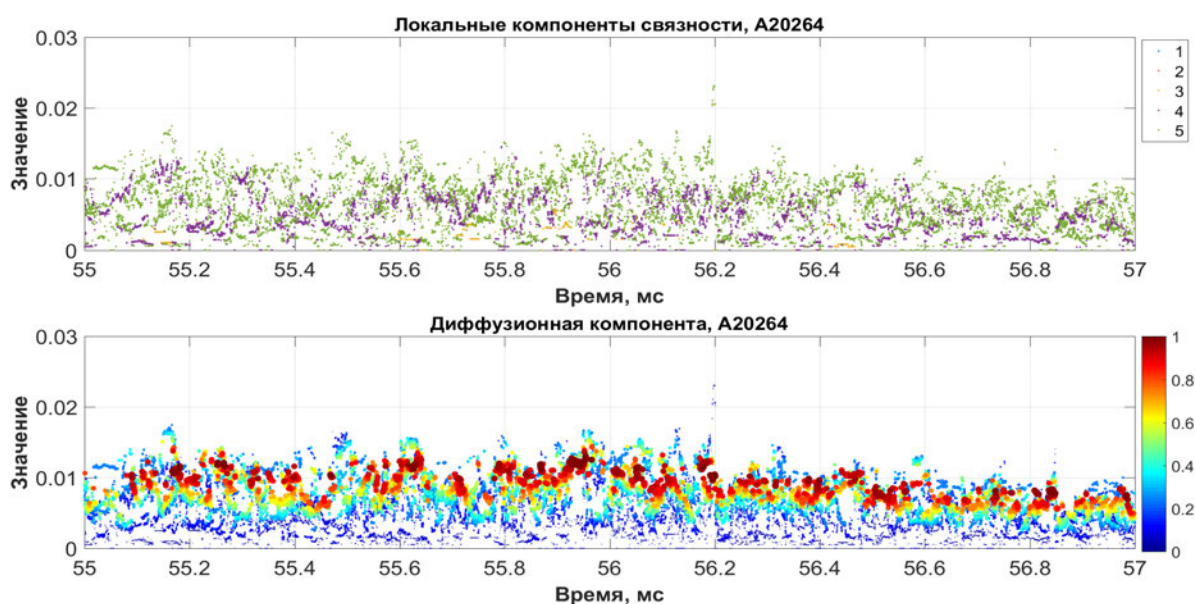
Рис. 5.15. Ансамбль A20264, диффузионная компонента (55–57 мс)
