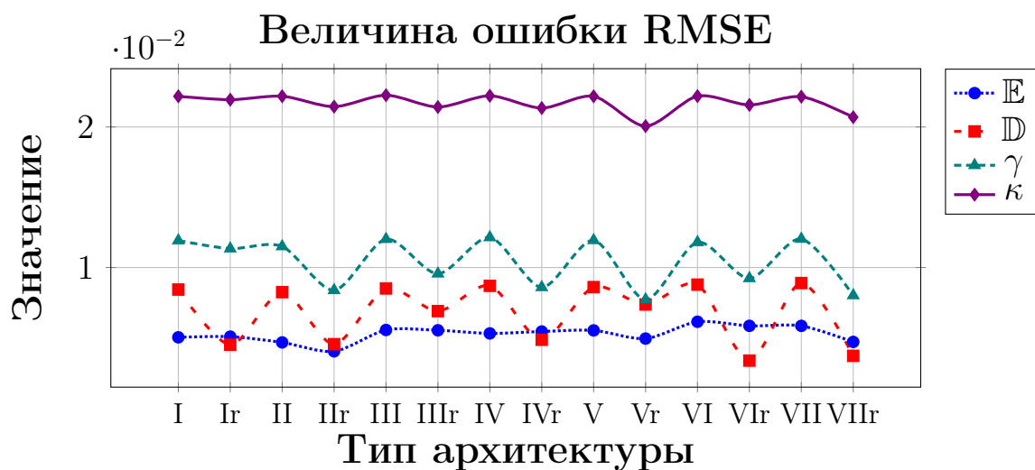
Рис. 5.26. Сравнение величины среднеквадратичных ошибок
