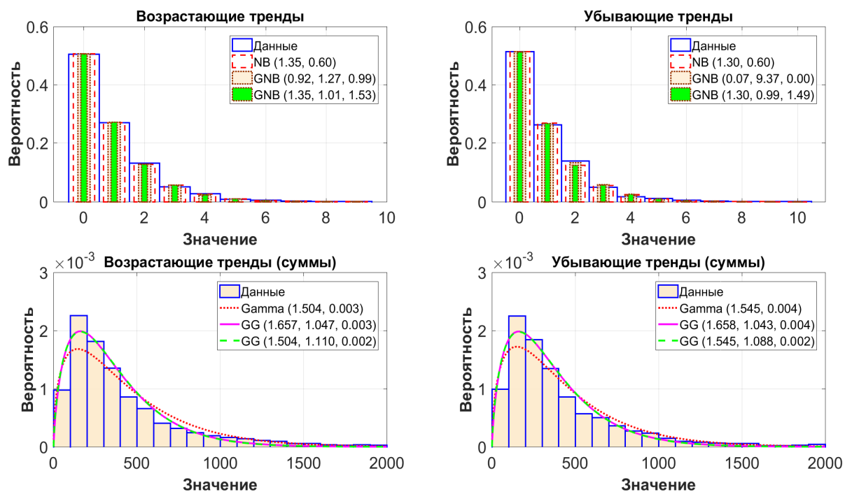
Рис. 6.70. Распределения характеристик (тропики, явные потоки)
