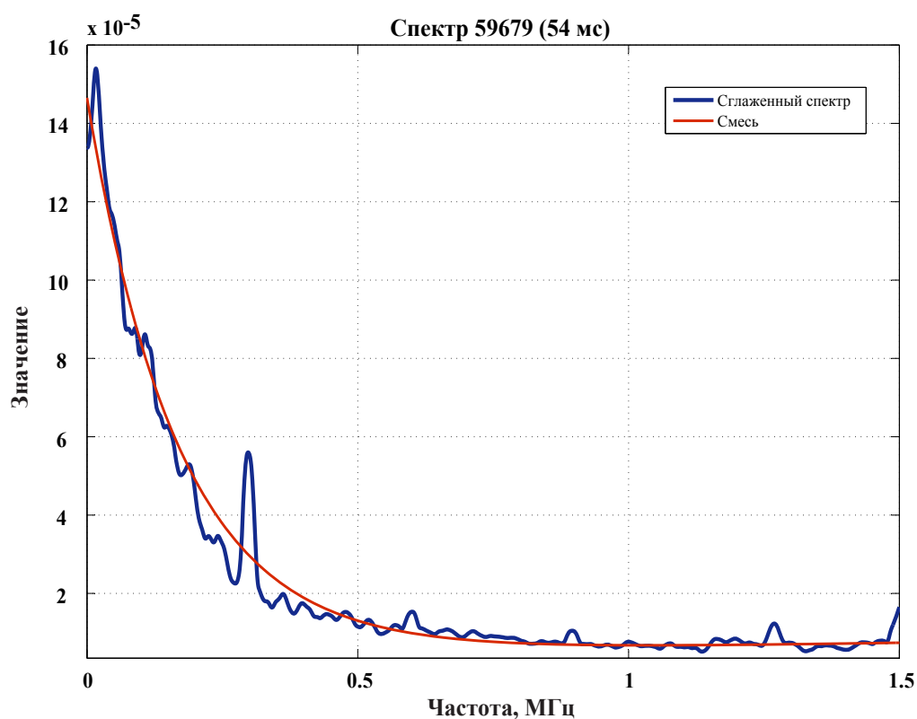
Рис. 5.5. Аппроксимация спектра 59679 (54 мс), гамма-распределения
