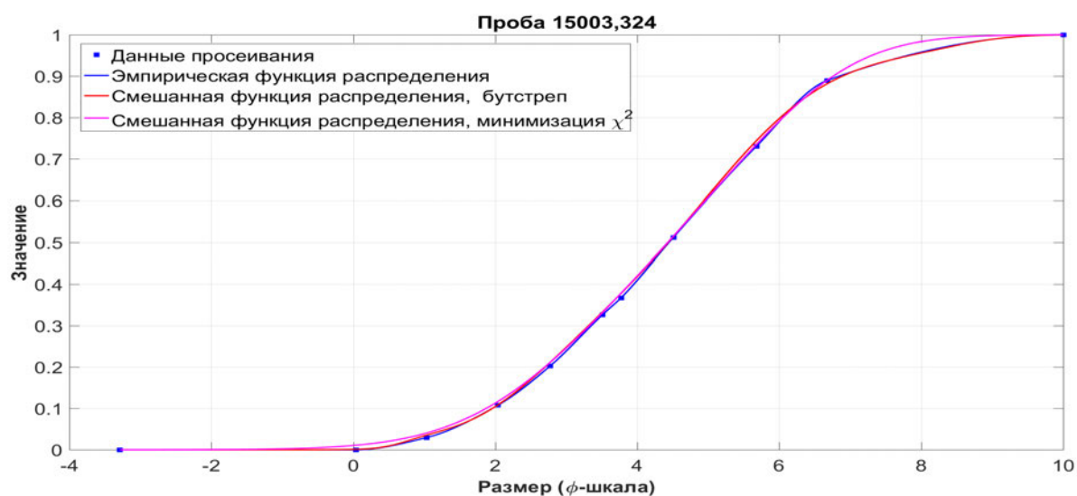
Рис. 4.14. Проба лунного грунта 15003,324 (миссия «Аполлон-15»)
