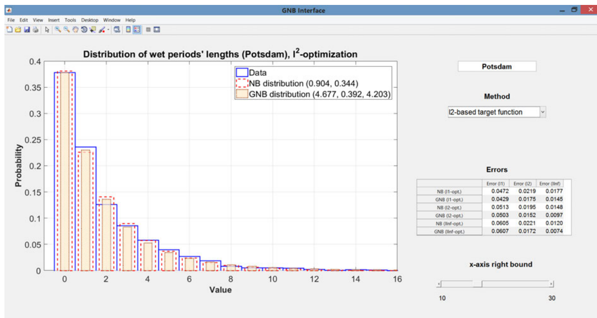
Рис. 7.11. Аппроксимация распределения длительностей дождливых периодов на основе метрики \ell^2
