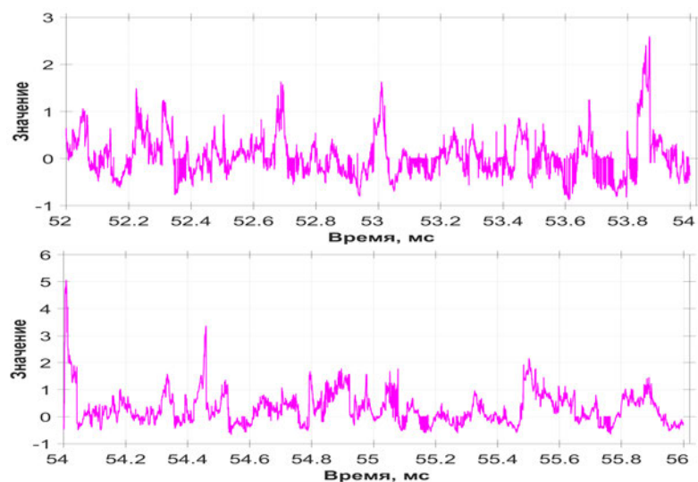
Рис. 5.18. Коэффициенты эксцесса для интервалов 52–54 мс и 54–56 мс
