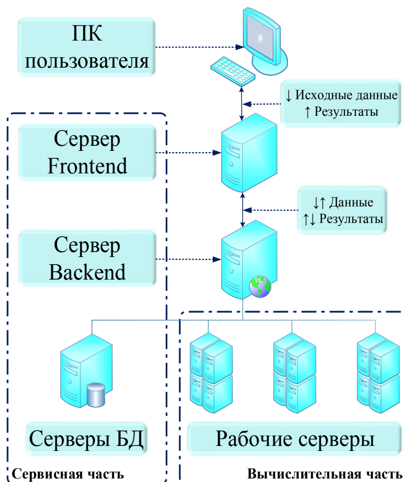
Рис. 7.17. Архитектура онлайн-сервиса и диаграмма потоков данных
