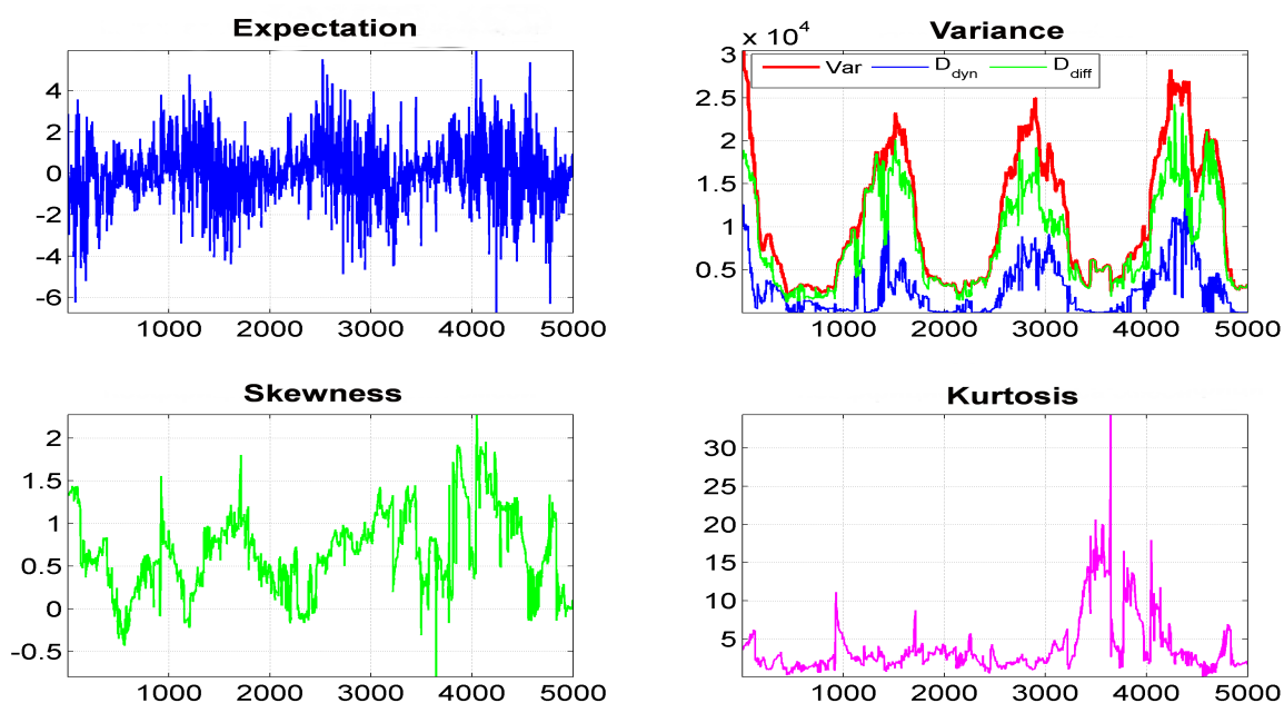
Рис. 6.53. Моментные характеристики
