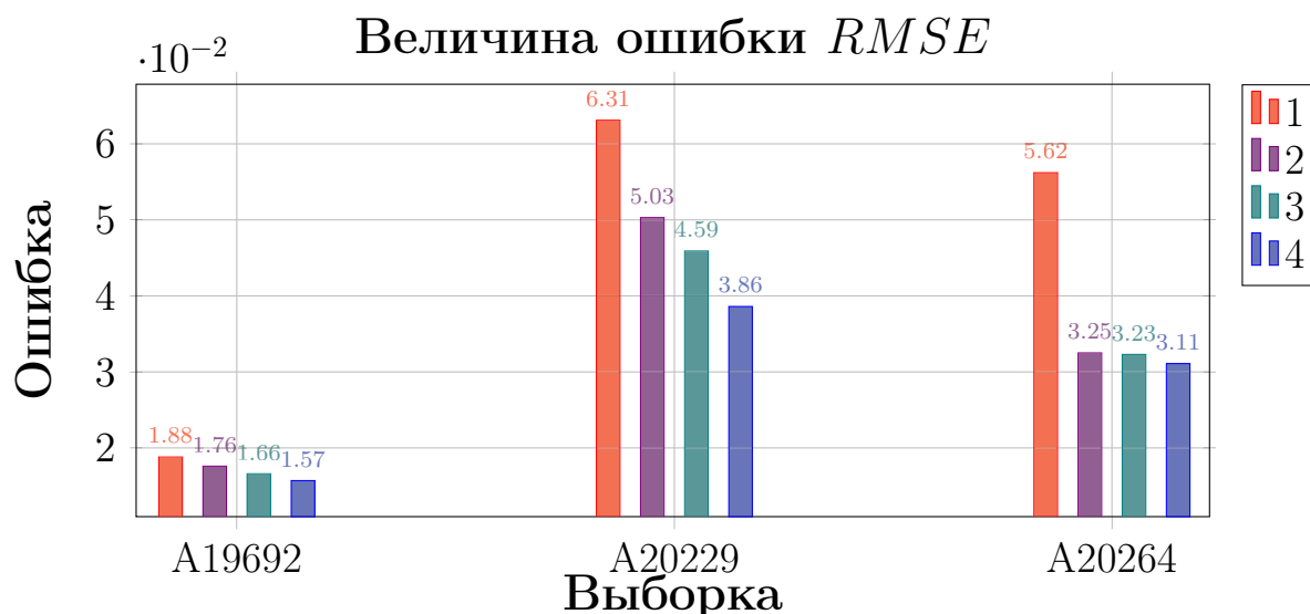
Рис. 5.24. Точность нейросетевых прогнозов исходных данных (1) и с расширенными обучающими наборами: выборочные (2), модельные моменты (3) и моменты смесей для приращений (4)
