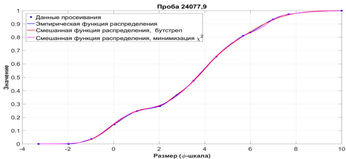
Рис. 4.16. Проба лунного грунта 24077,9 (миссия «Луна-24»)
