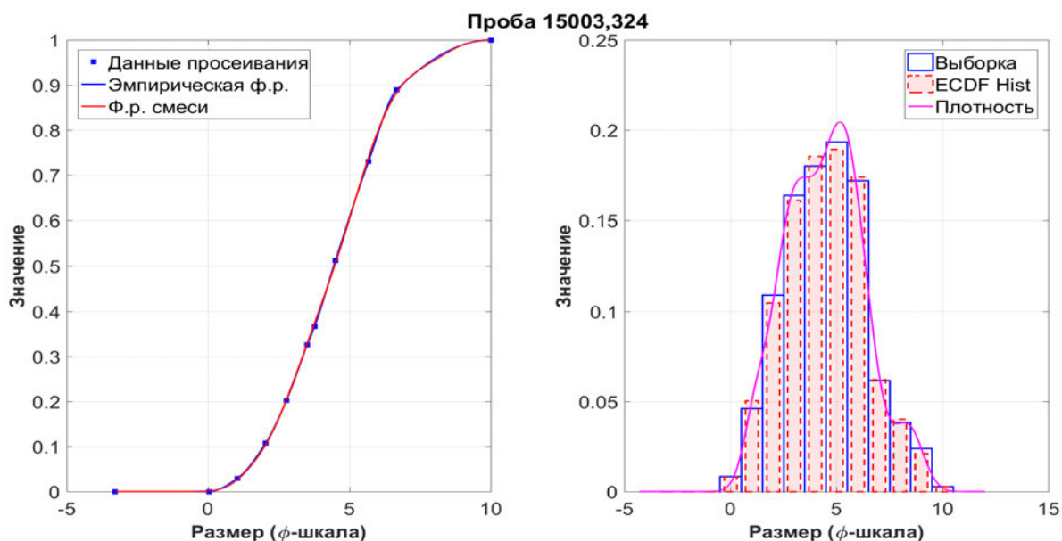
Рис. 4.4. Проба лунного грунта 15003,324 (миссия «Аполлон-15»)
