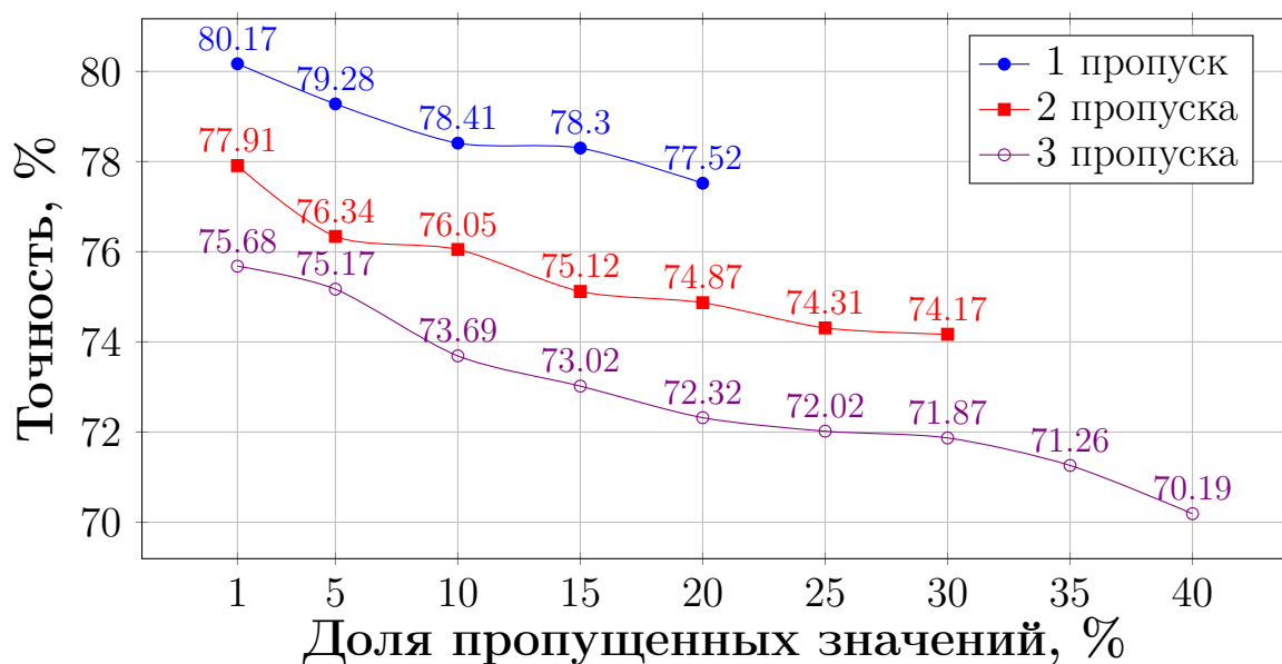
Рис. 6.11. Заполнение пропусков с использованием SVM, Потсдам
