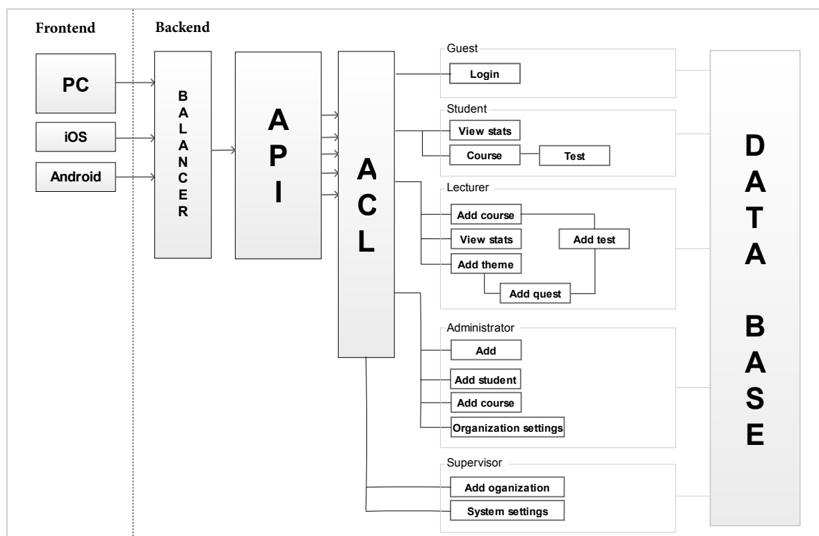
Рис. 7.20. Архитектура системы управления обучением научно-образовательной цифровой платформы ФИЦ ИУ РАН
