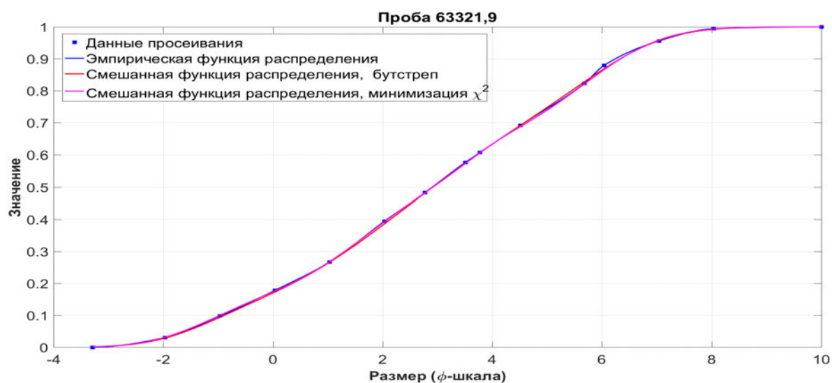
Рис. 4.17. Проба лунного грунта 63321,9 (миссия «Аполлон-16»)
