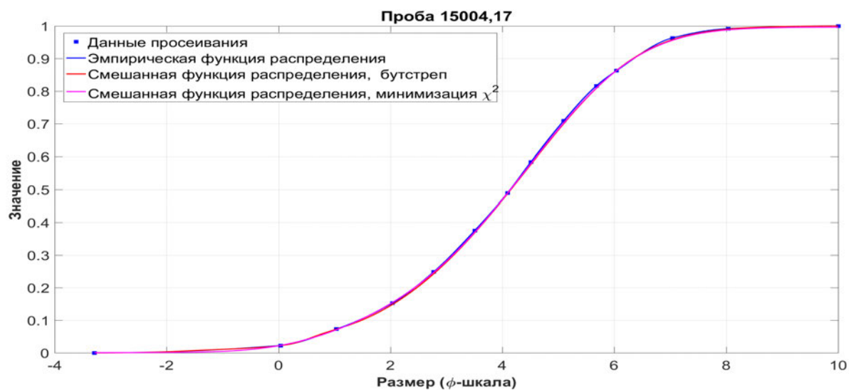
Рис. 4.15. Проба лунного грунта 15004,17 (миссия «Аполлон-15»)
