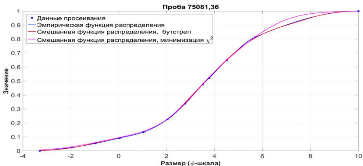
Рис. 4.19. Проба лунного грунта 75081,36 (миссия «Аполлон-17»)
