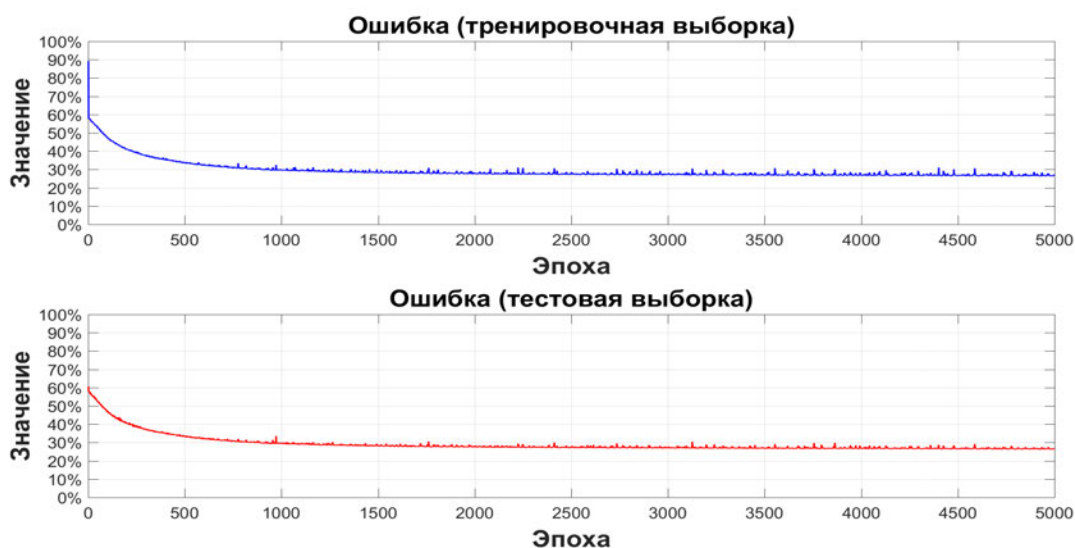
Рис. 6.7. Ошибки для двухдневного прогноза, Потсдам
