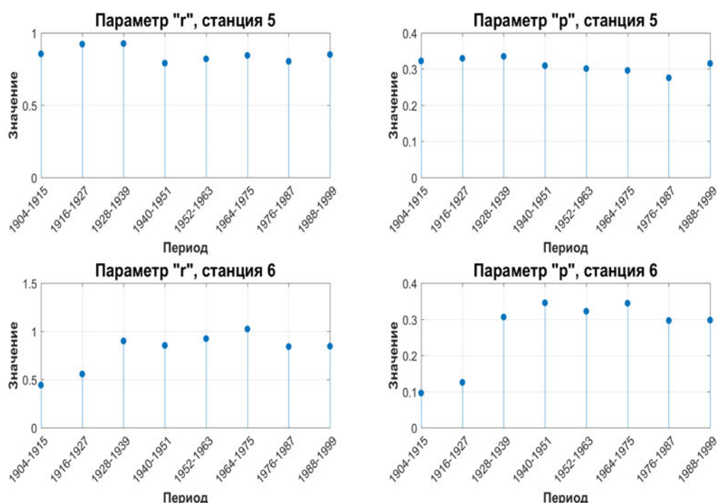
Рис. 6.19. «Дождливые» периоды, станции 5 и 6, окно 12 лет
