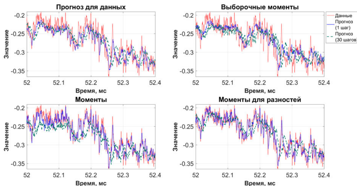
Рис. 5.20. Пример прогноза для ряда A19692 (52,00–52,40 мс)
