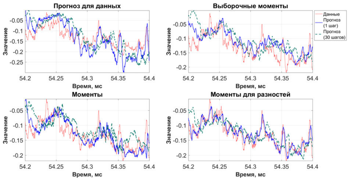
Рис. 5.22. Пример прогноза для ряда A20229 (54,20–54,40 мс)
