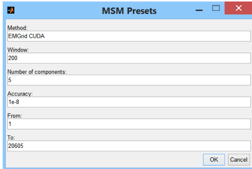
Рис. 7.2. Пример: настройки параметров СРС-метода
