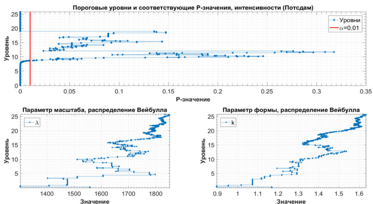
Рис. 6.40. Пороговые уровни и соответствующие P -значения, Потсдам
