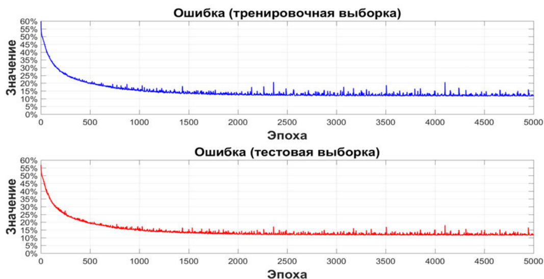
Рис. 6.4. Ошибки для двухдневного прогноза, Потсдам
