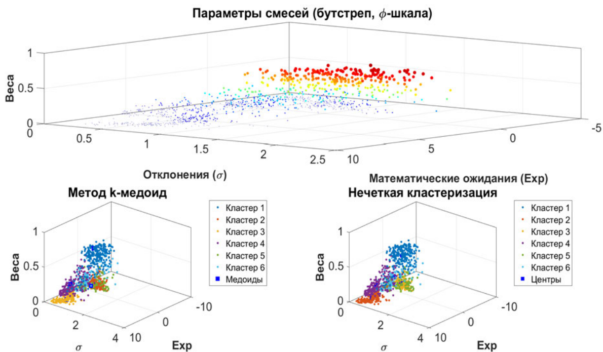
Рис. 4.25. Кластеризация параметров в пространстве (бутстреп, \phi -шкала)
