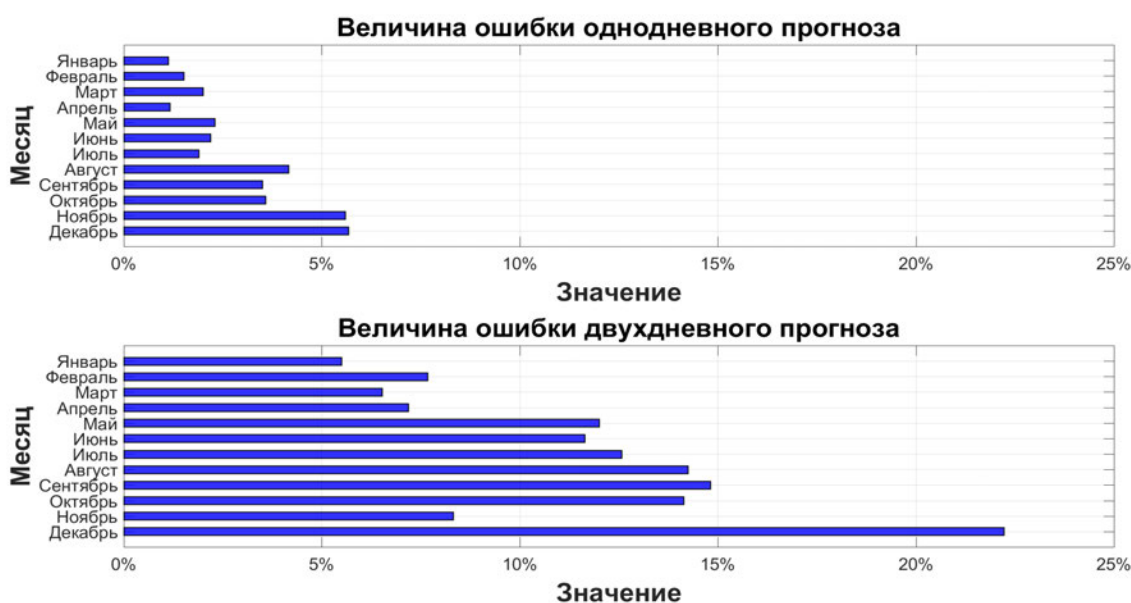
Рис. 6.5. Величины ошибок с учетом сезонного фактора, Потсдам
