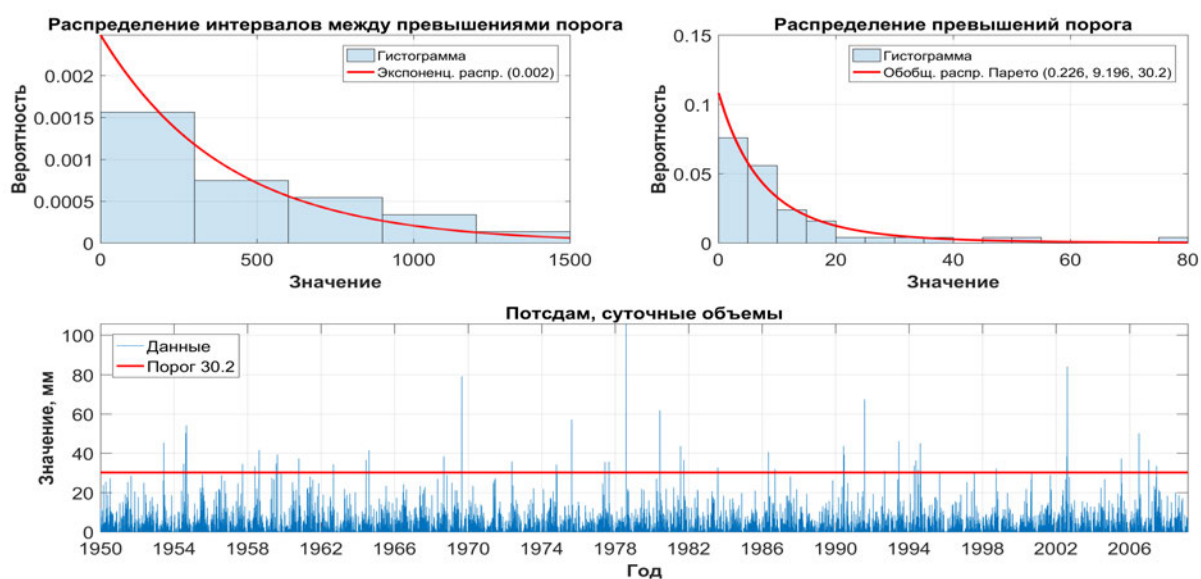
Рис. 6.30. Пороговый уровень для суточных объемов осадков, Потсдам
