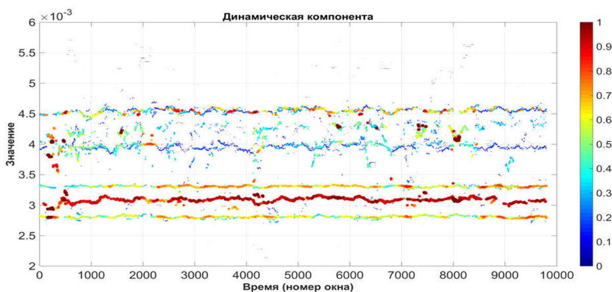
Рис. 3.23. Динамическая компонента после удаления шума
