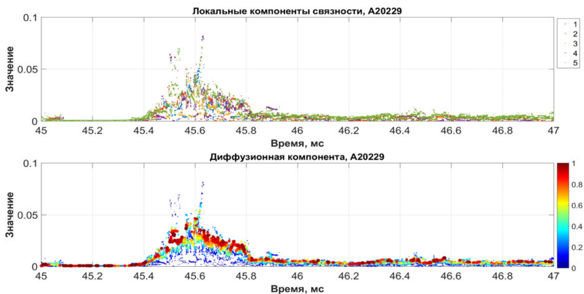
Рис. 5.9. Ансамбль A20229, диффузионная компонента (45–47 мс)
