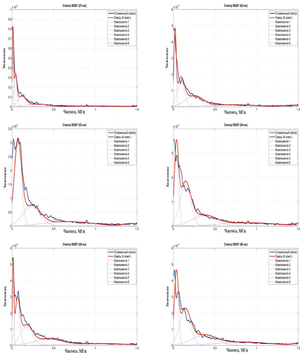
Рис. 5.2. Аппроксимация спектра 59287 с 51 мс по 56 мс
