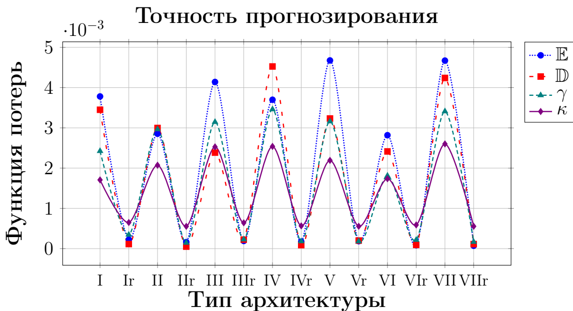
Рис. 5.27. Сравнение величины функции потерь
