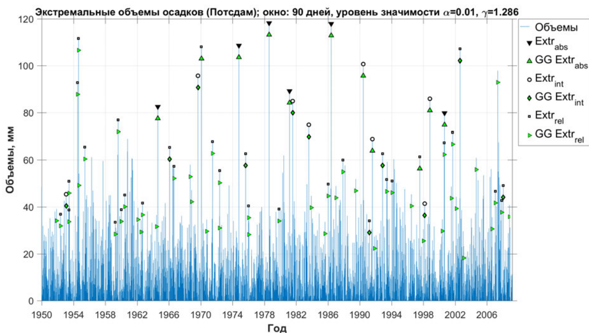
Рис. 6.36. Аномальные объемы осадков, окно 90 дней (Потсдам)
