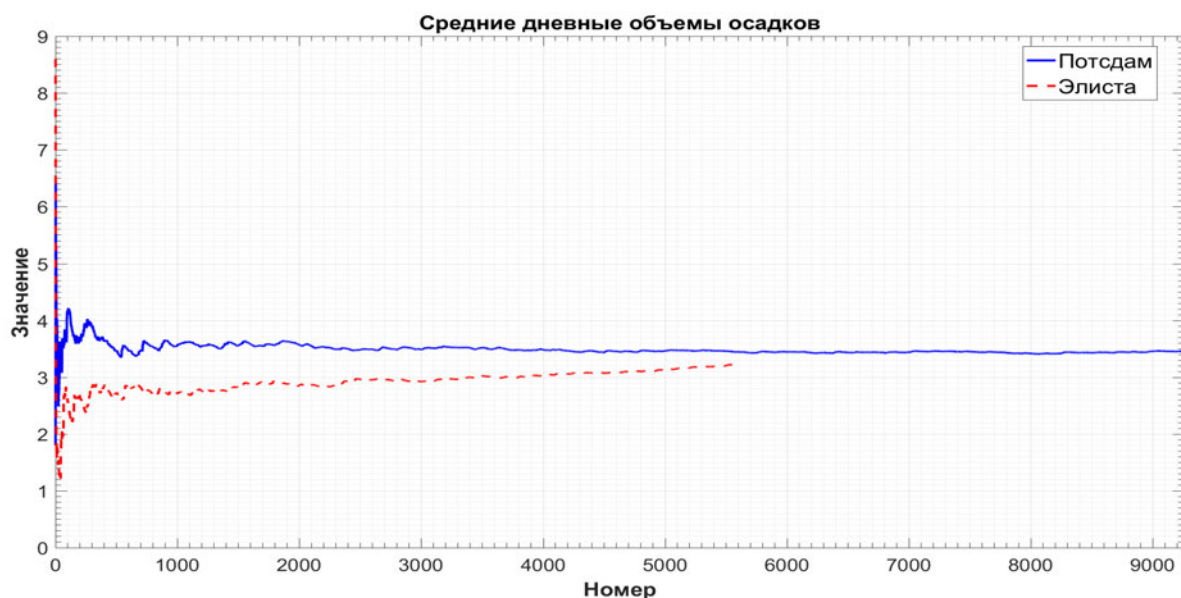
Рис. 6.28. Нарушение классического закона больших чисел для осадков
