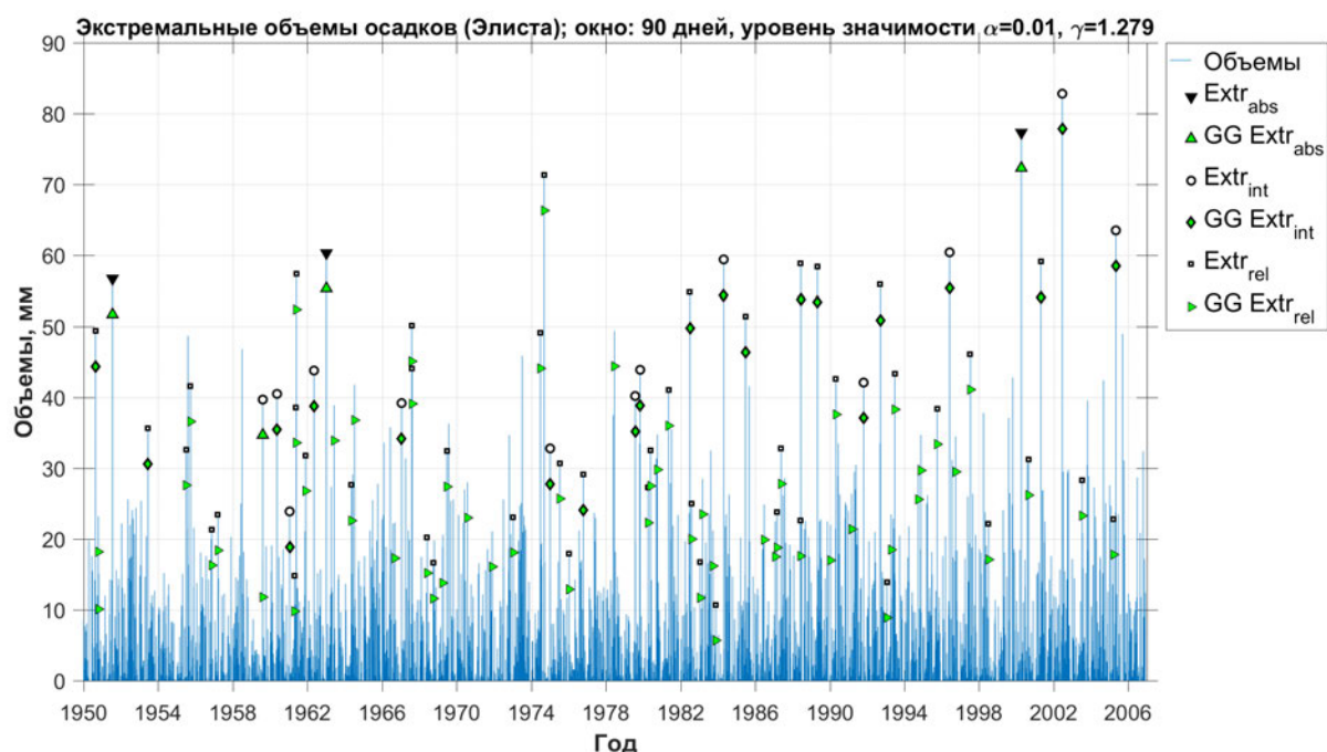
Рис. 6.38. Аномальные объемы осадков, окно 90 дней (Элиста)
