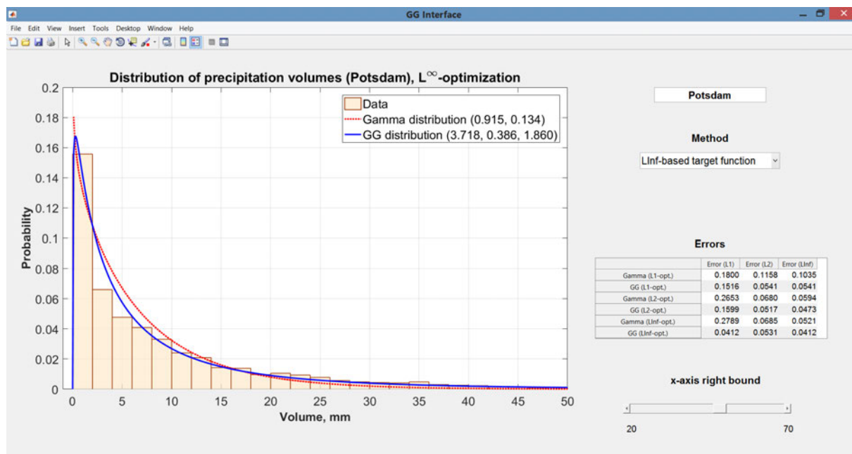
Рис. 7.15. Аппроксимация распределения объемов осадков за дождливые периоды на основе метрики L^\infty
