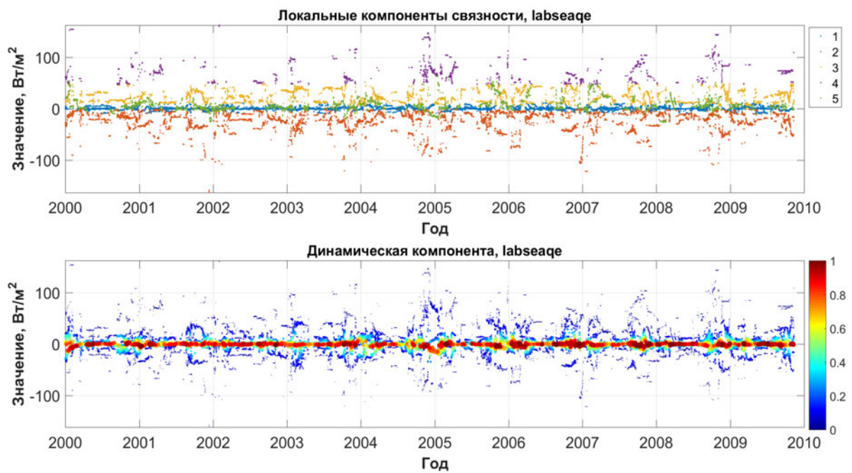
Рис. 6.58. Оценки распределения сдвига (Лабрадорское море, явные потоки)
