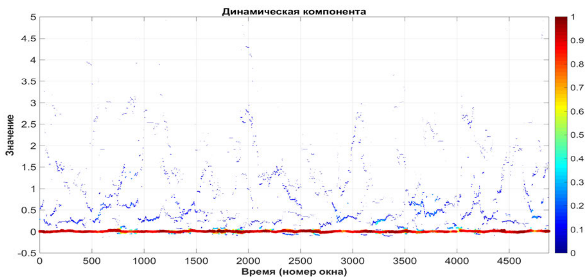
Рис. 3.14. Динамическая компонента модифицированной выборки
