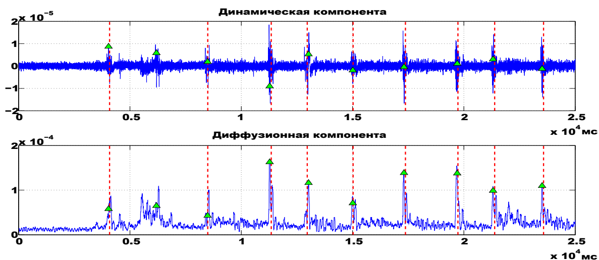
Рис. 3.7. Скользящее детектирование событий: прямое направление
