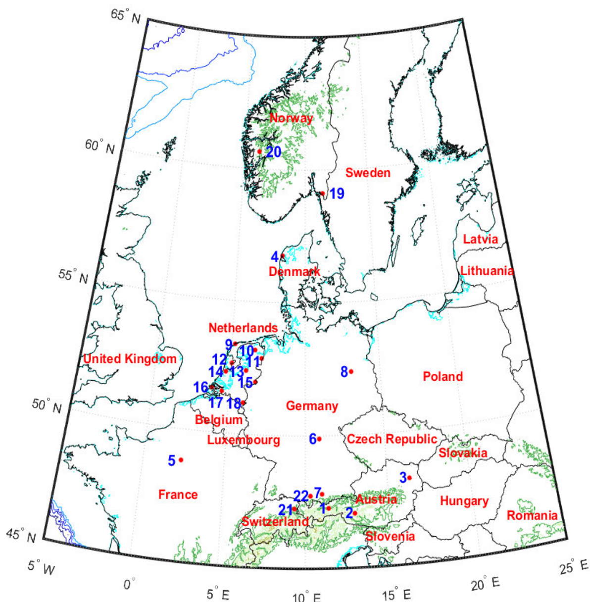
Рис. 6.9. Географическое расположение анализируемых станций
