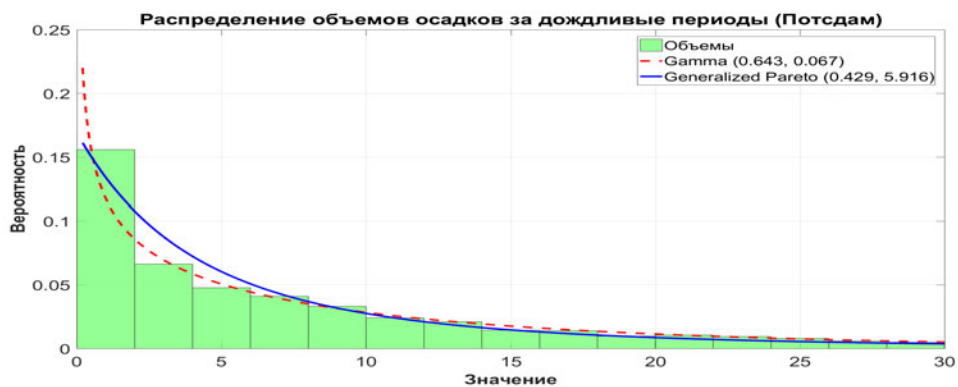
Рис. 6.22. Распределение объемов осадков за периоды, Потсдам
