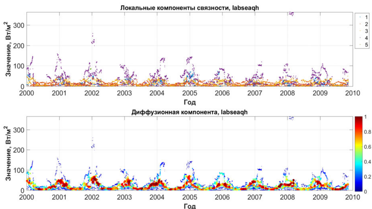
Рис. 6.61. Оценки распределения коэффициента диффузии (Лабрадорское море, скрытые потоки)
