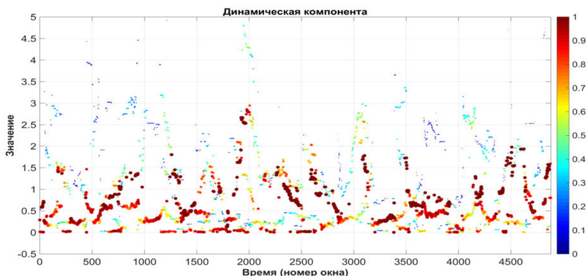
Рис. 3.16. Динамическая компонента исходных данных после удаления внесенного шума
