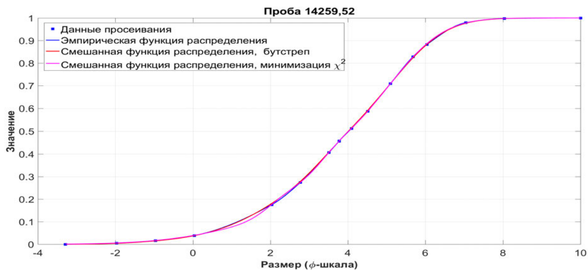
Рис. 4.13. Проба лунного грунта 14259,52 (миссия «Аполлон-14»)
