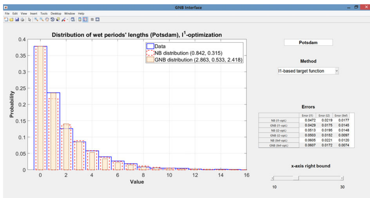
Рис. 7.10. Аппроксимация распределения длительностей дождливых периодов на основе метрики \ell^1
