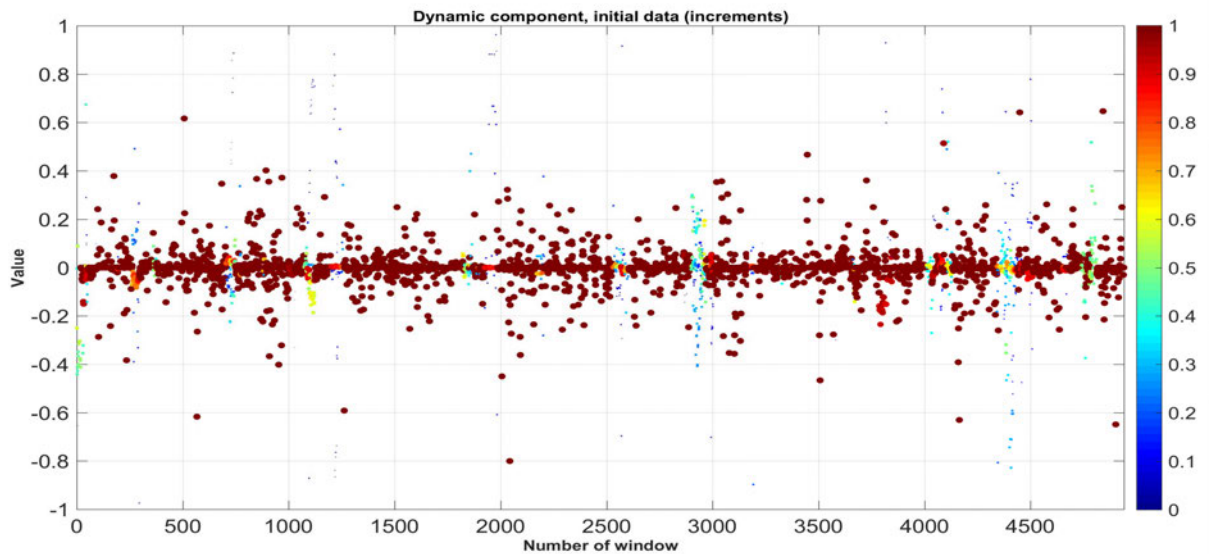
Рис. 3.18. Динамическая компонента для приращений исходных данных
