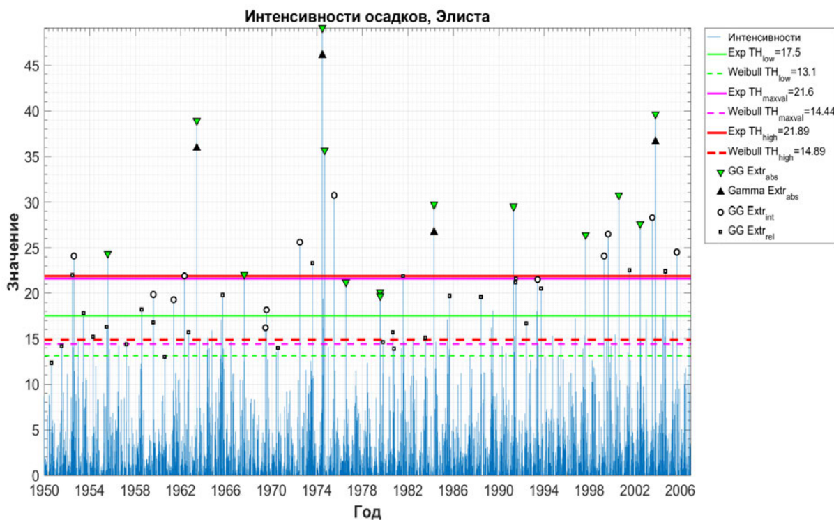
Рис. 6.43. Аномальные интенсивности осадков, окно 365 дней (Элиста)
