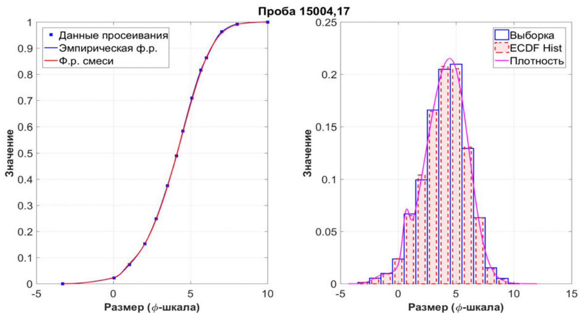
Рис. 4.5. Проба лунного грунта 15004,17 (миссия «Аполлон-15»)
