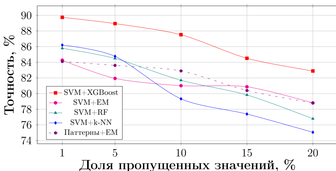
Рис. 6.12. Точность гибридных методов, 1 пропуск (Потсдам)
