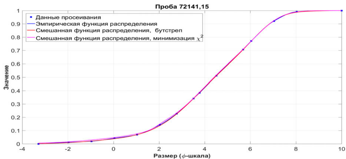
Рис. 4.18. Проба лунного грунта 72141,15 (миссия «Аполлон-17»)
