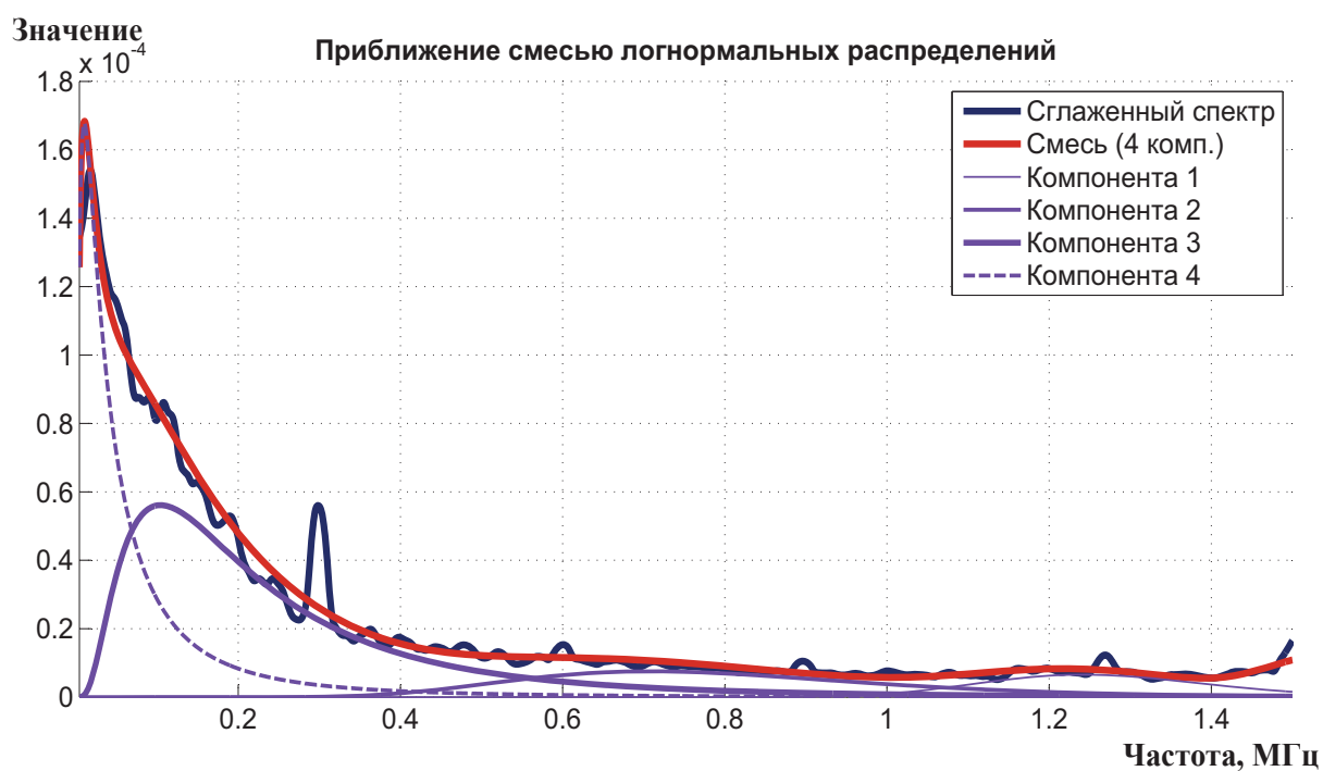
Рис. 5.6. Аппроксимация спектра 59679 (54 мс), логнормальные смеси
