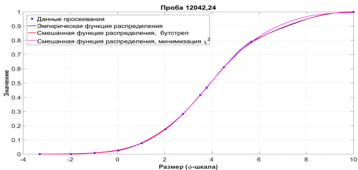
Рис. 4.11. Проба лунного грунта 12042,24 (миссия «Апполон-12»)
