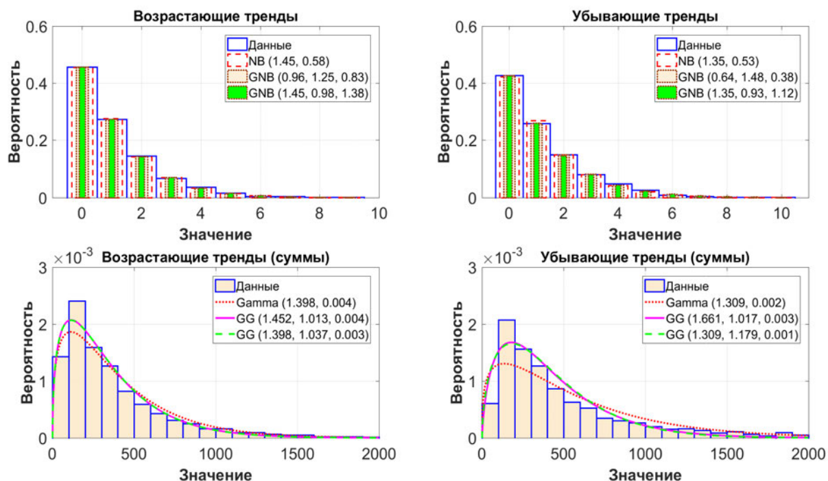
Рис. 6.68. Распределения характеристик (Гольфстрим, явные потоки)
