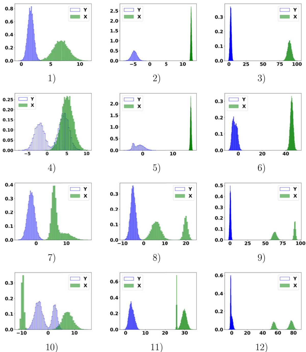
Рис. 3.2. Тестовые данные для сигнала и шума (выборки 1 – 12)
