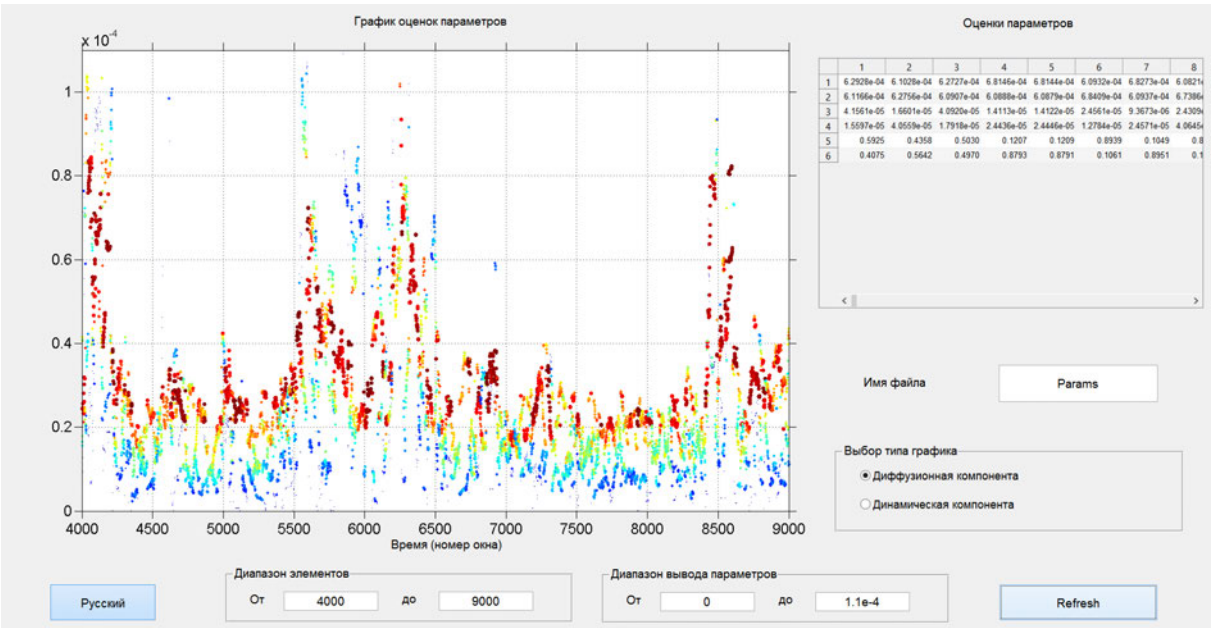
Рис. 7.6. Пример: диффузионная компонента
