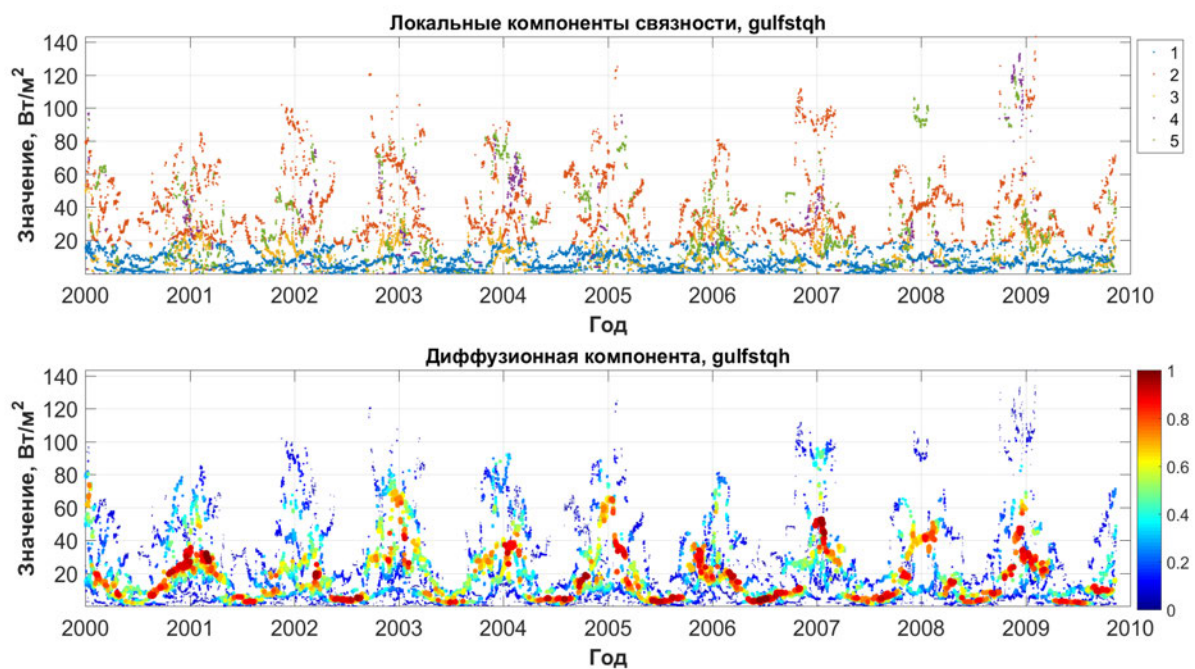
Рис. 6.57. Оценки распределения коэффициента диффузии (Гольфстрим, скрытые потоки)
