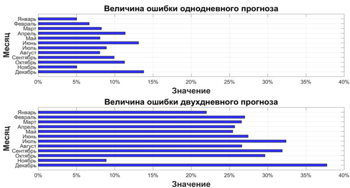
Рис. 6.8. Величины ошибок с учетом сезонного фактора, Потсдам
