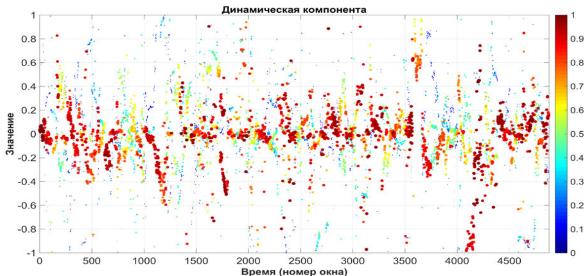
Рис. 3.19. Динамическая компонента для приращений после модификации исходных данных
