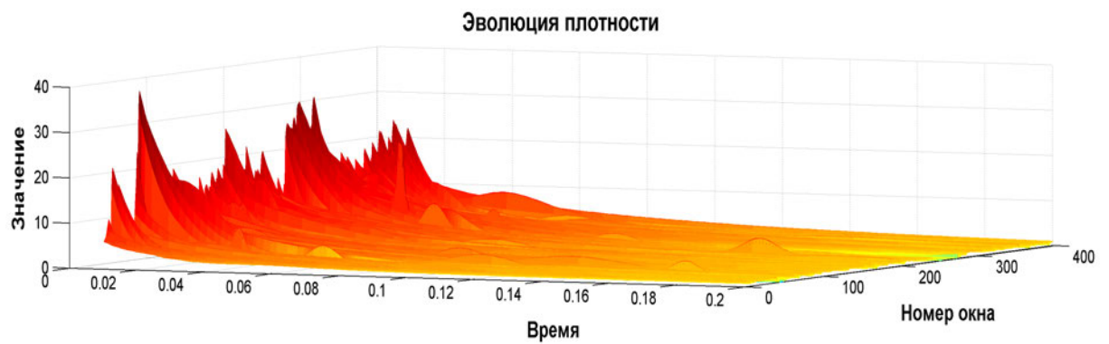
Рис. 2.1. Эволюция плотности смеси гамма-распределений
