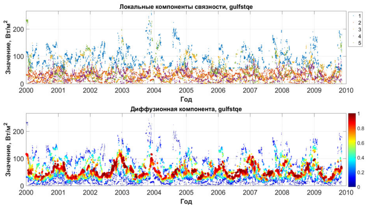
Рис. 6.56. Оценки распределения коэффициента диффузии (Гольфстрим, явные потоки)
