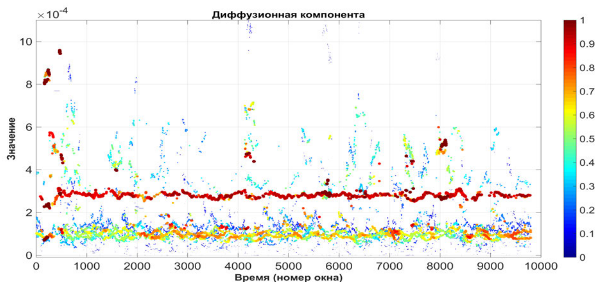
Рис. 3.24. Диффузионная компонента после удаления шума
