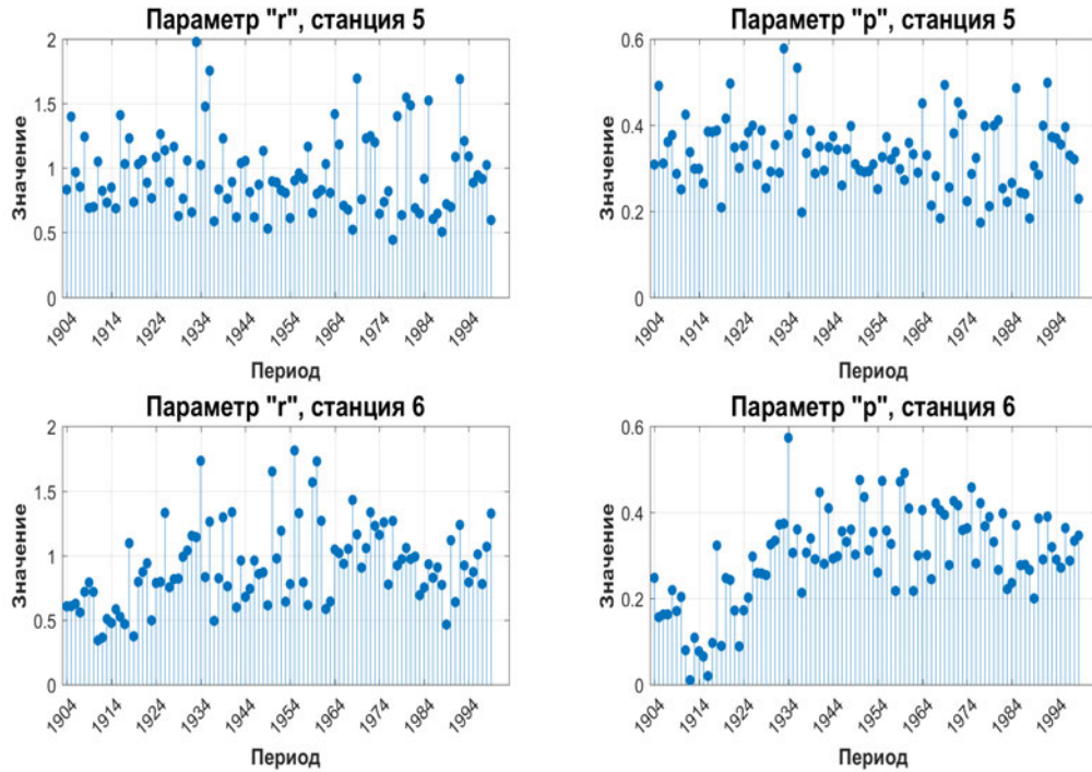
Рис. 6.16. «Дождливые» периоды, станции 5 и 6, окно 1 год
