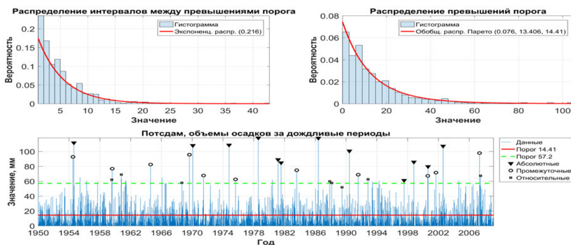
Рис. 6.34. Сравнение методов определения экстремальности, Потсдам
