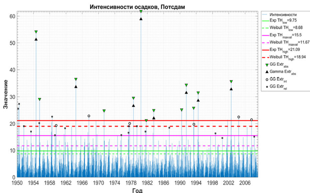
Рис. 6.42. Аномальные интенсивности осадков, окно 365 дней (Потсдам)
