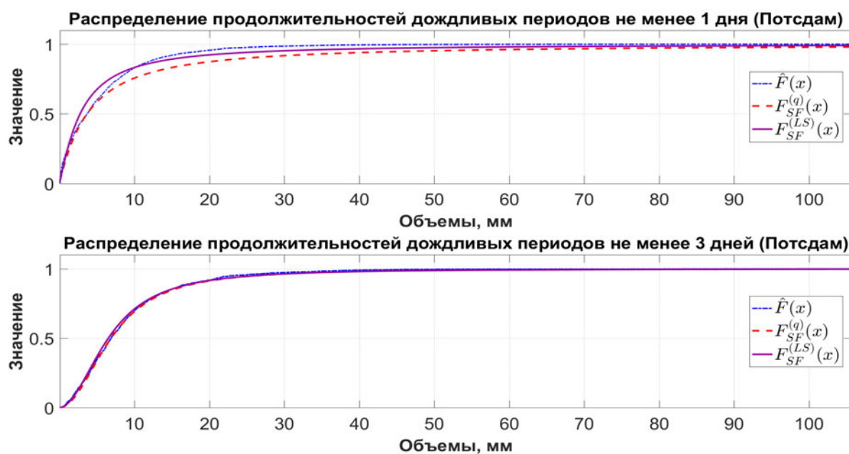
Рис. 6.44. Аппроксимация асимптотическим распределением, Потсдам
