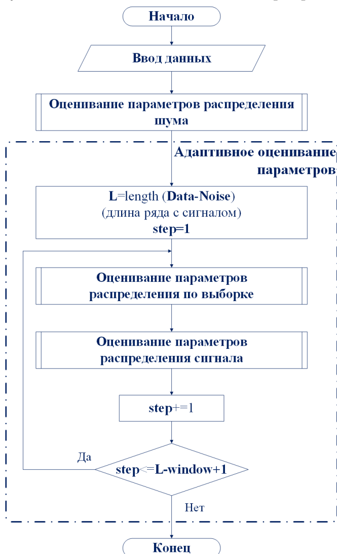
Рис. 3.1. Алгоритм адаптивного определения параметров распределения сигнала с помощью СРС-метода
