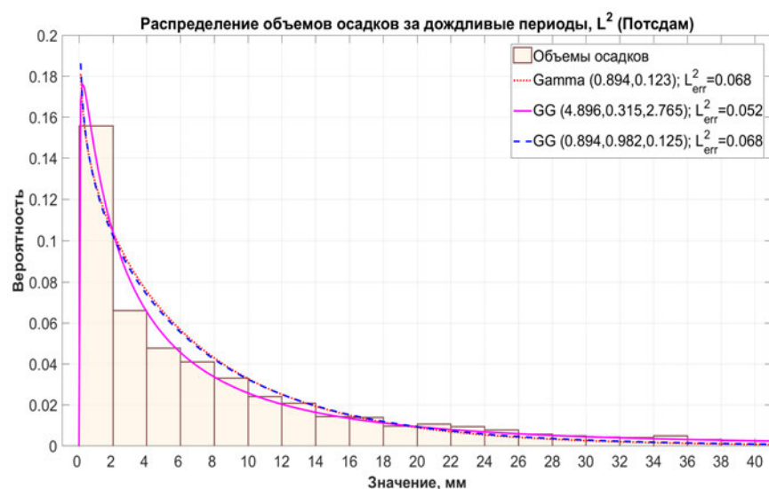
Рис. 6.26. Распределение объемов осадков за «дождливые» периоды в Потсдаме, пример аппроксимации в L^2
