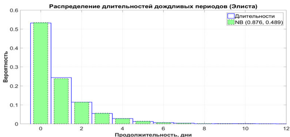
Рис. 6.15. Распределение длительностей периодов, Элиста
