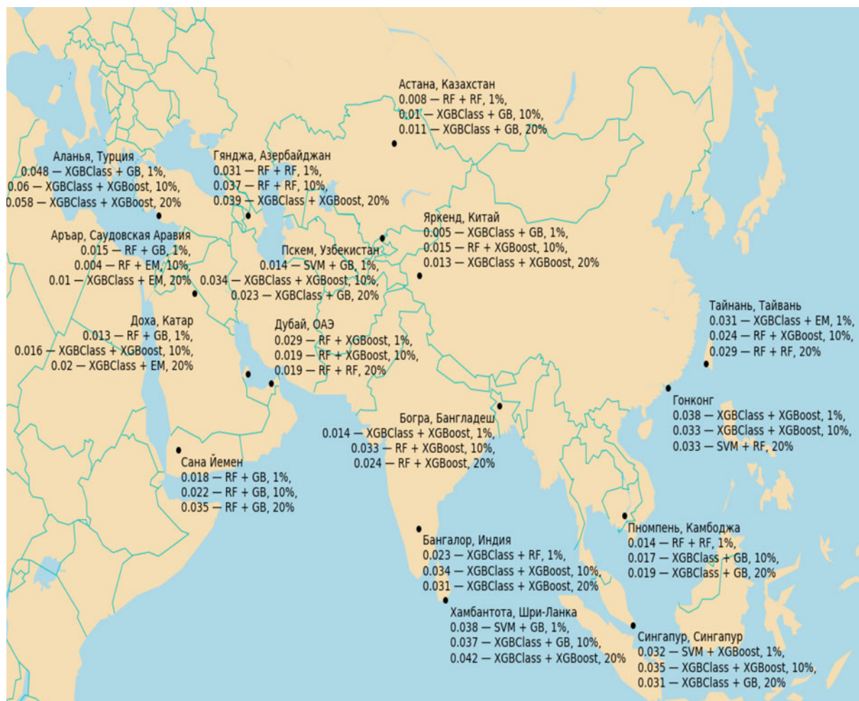
Рис. 6.13. Метеостанции и точность заполнения пропусков
