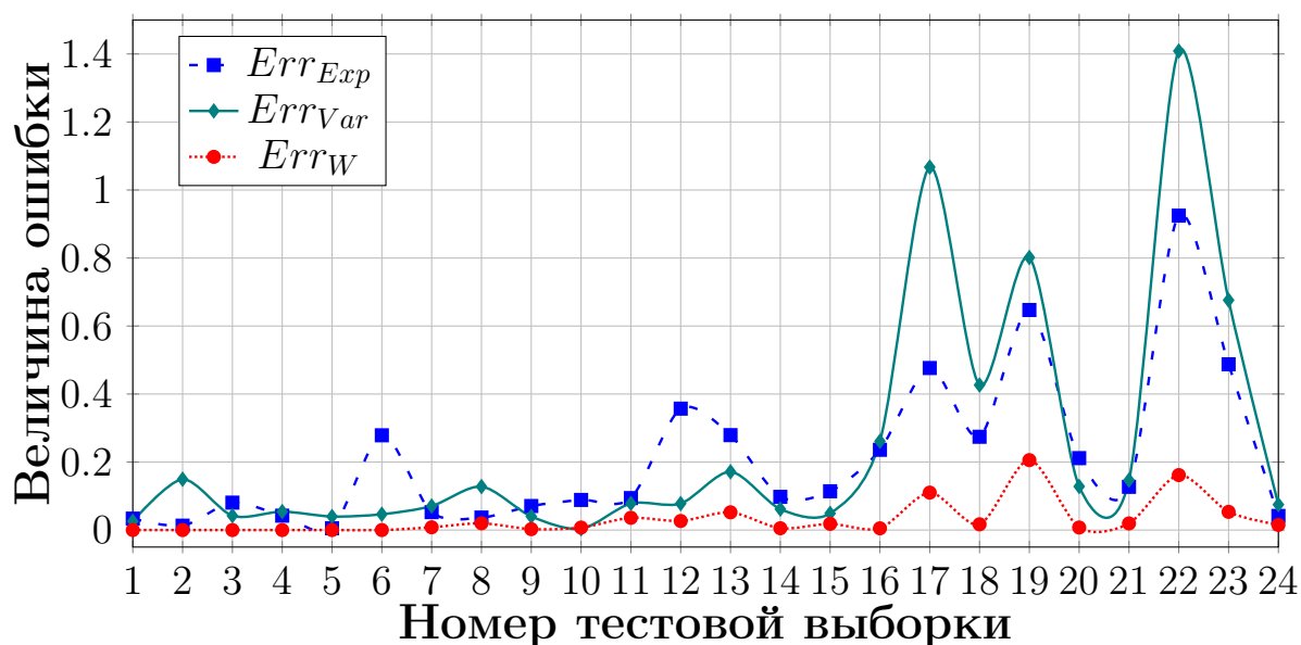
Рис. 3.5. Величины вычислительных ошибок для математических ожиданий ( Err_{Exp} ), дисперсий ( Err_{Var} ) и весов ( Err_W )
