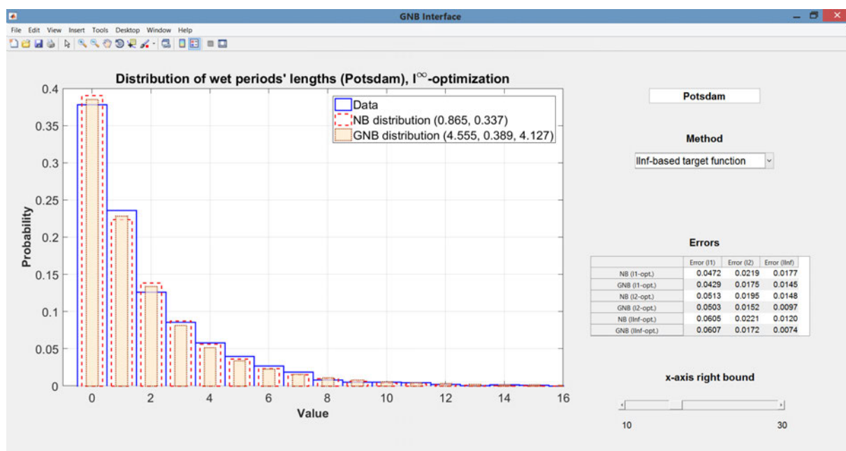
Рис. 7.12. Аппроксимация распределения длительностей дождливых периодов на основе метрики \ell^\infty
