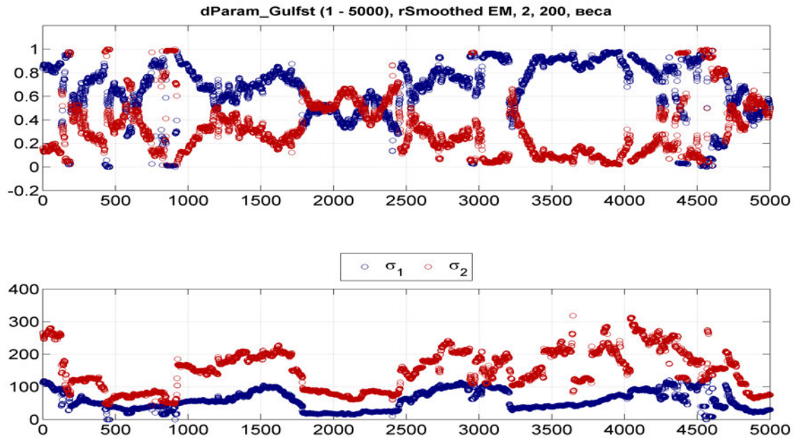
Рис. 6.66. Определение доли экстремальных наблюдений
