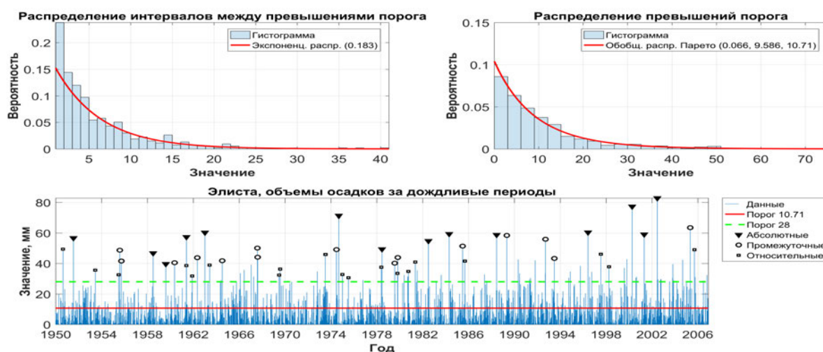
Рис. 6.35. Сравнение методов определения экстремальности, Элиста
