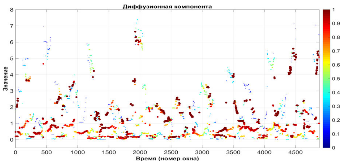
Рис. 3.17. Диффузионная компонента исходных данных после удаления внесенного шума
