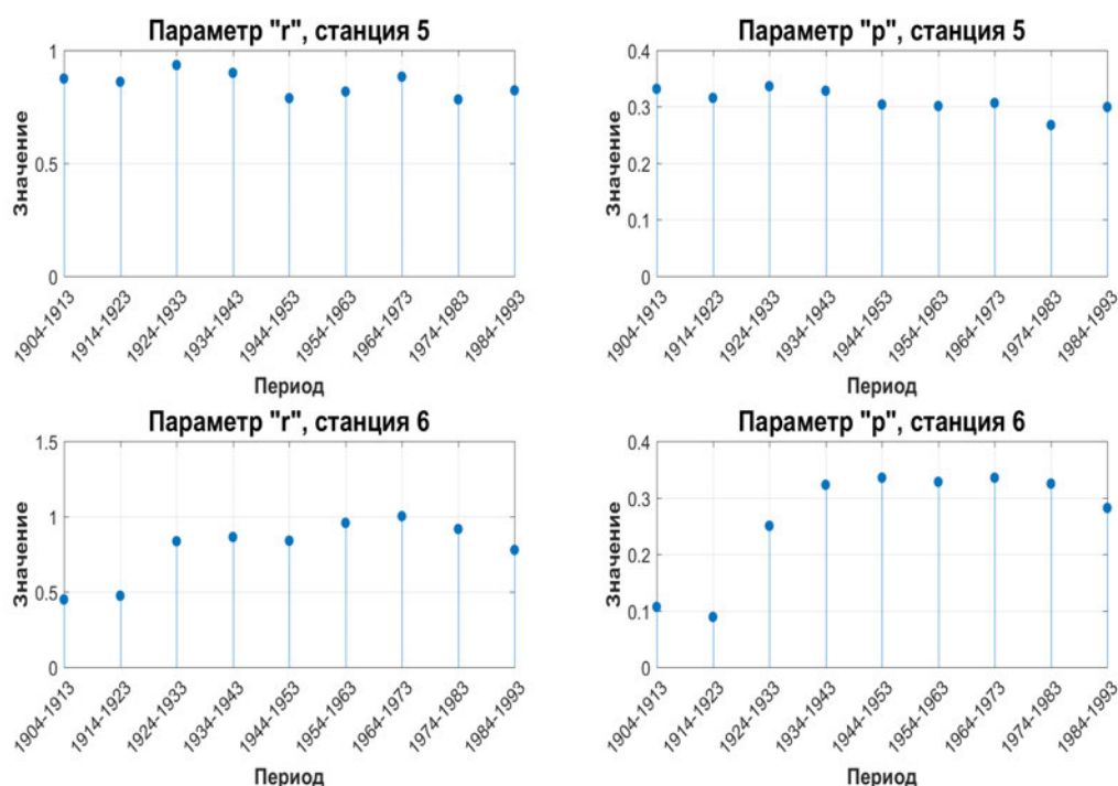
Рис. 6.18. «Дождливые» периоды, станции 5 и 6, окно 10 лет
