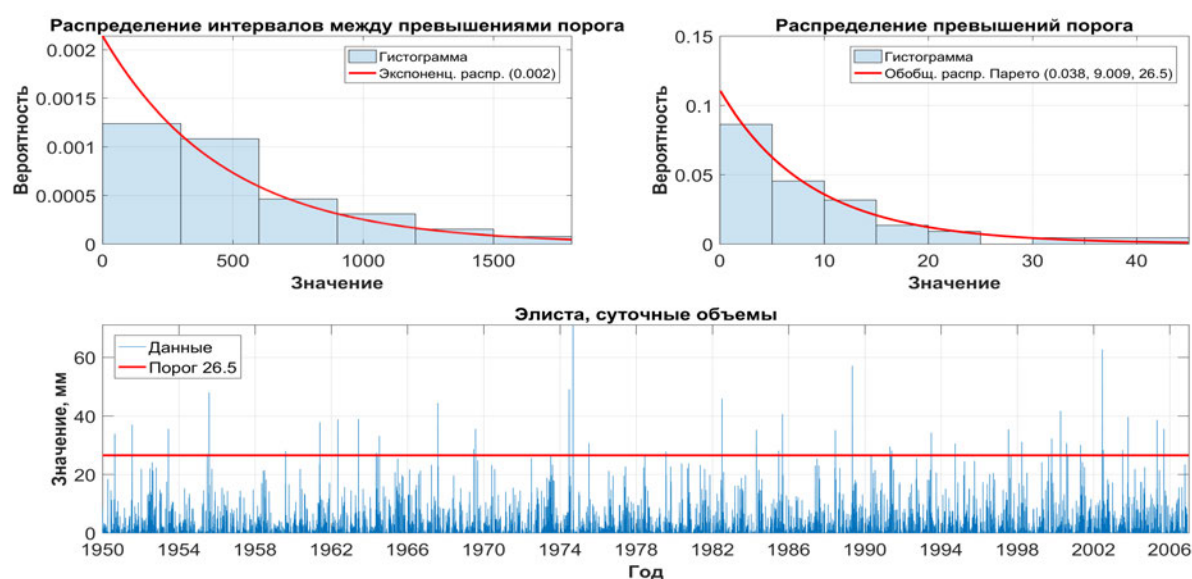
Рис. 6.31. Пороговый уровень для суточных объемов осадков, Элиста
