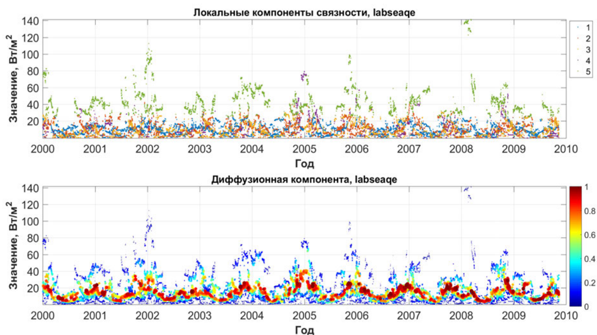
Рис. 6.60. Оценки распределения коэффициента диффузии (Лабрадорское море, явные потоки)
