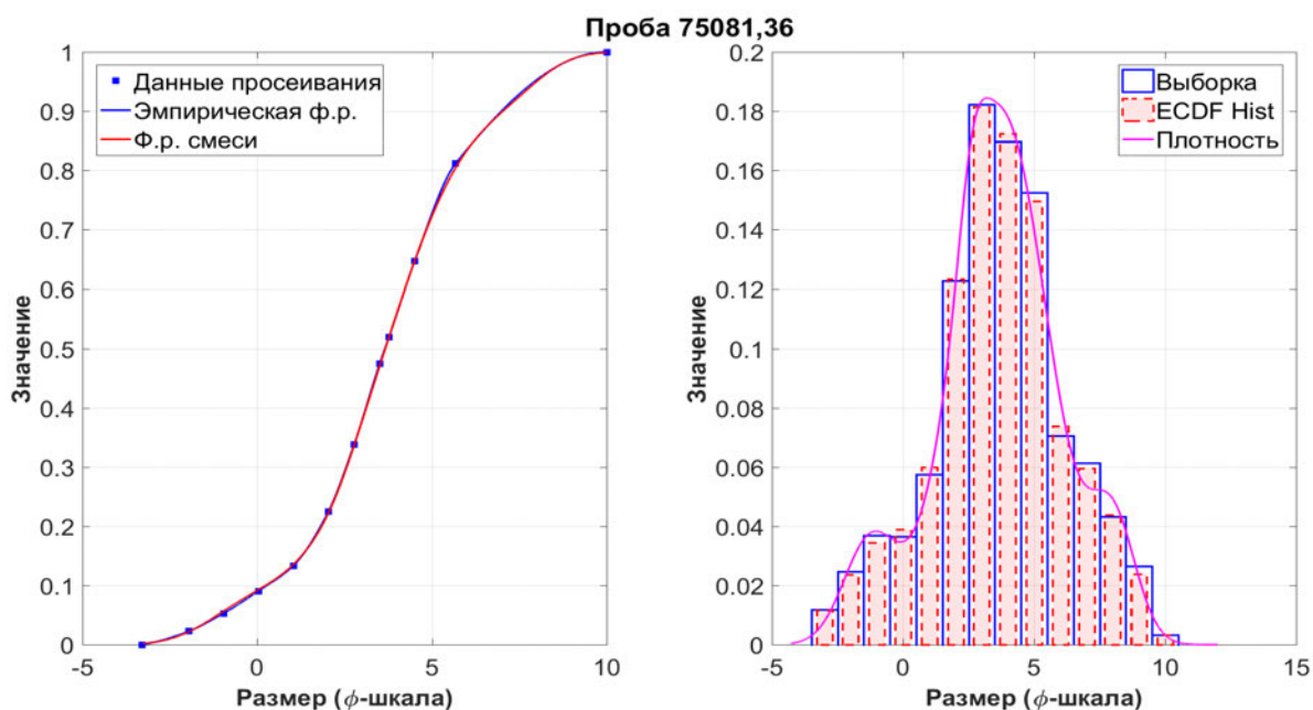
Рис. 4.9. Проба лунного грунта 75081,36 (миссия «Аполлон-17»)
