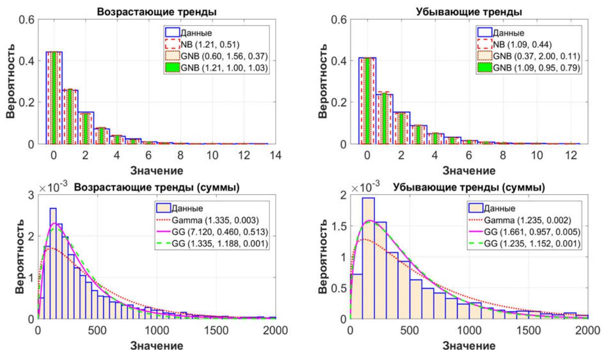
Рис. 6.69. Распределения характеристик (Гольфстрим, скрытые потоки)
