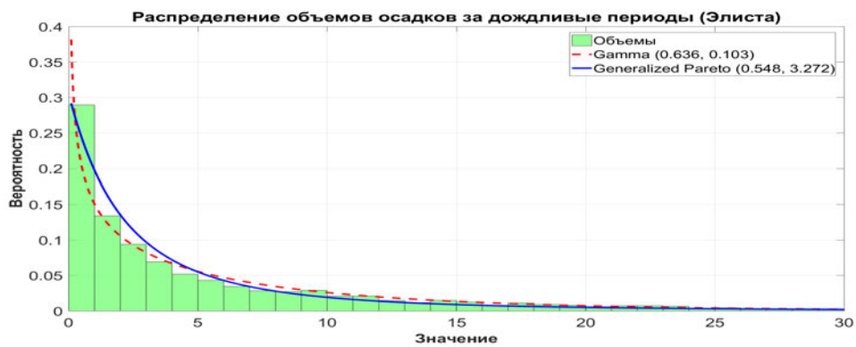
Рис. 6.23. Распределение объемов осадков за периоды, Элиста
