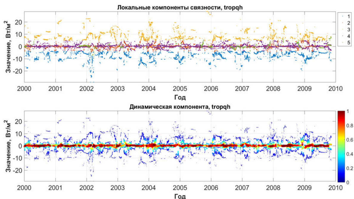
Рис. 6.63. Оценки распределения сдвига (тропики, скрытые потоки)
