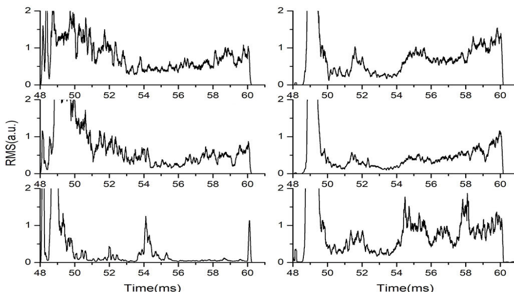
Рис. 5.16. Временная эволюция плотности флуктуаций (графики слева) и приращений (справа)
