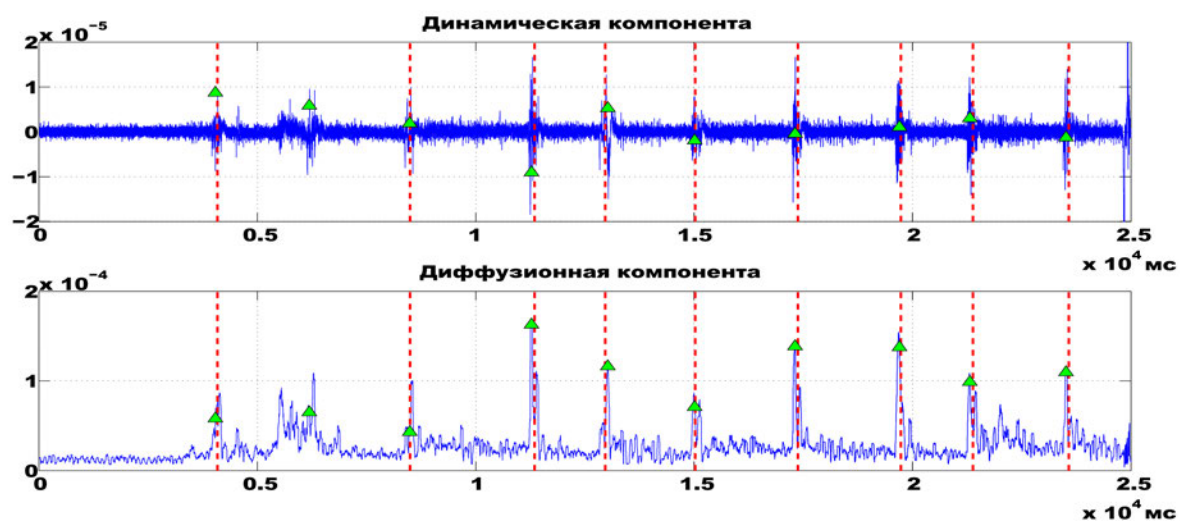
Рис. 3.8. Скользящее детектирования событий: обратное направление
