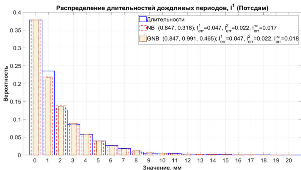
Рис. 6.24. Распределение длительностей «дождливых» периодов в Потсдаме, пример аппроксимации в \ell^1
