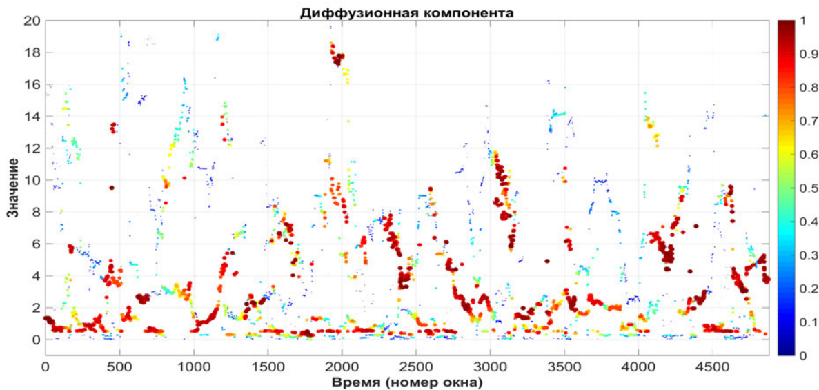
Рис. 3.20. Диффузионная компонента для приращений исходных данных
