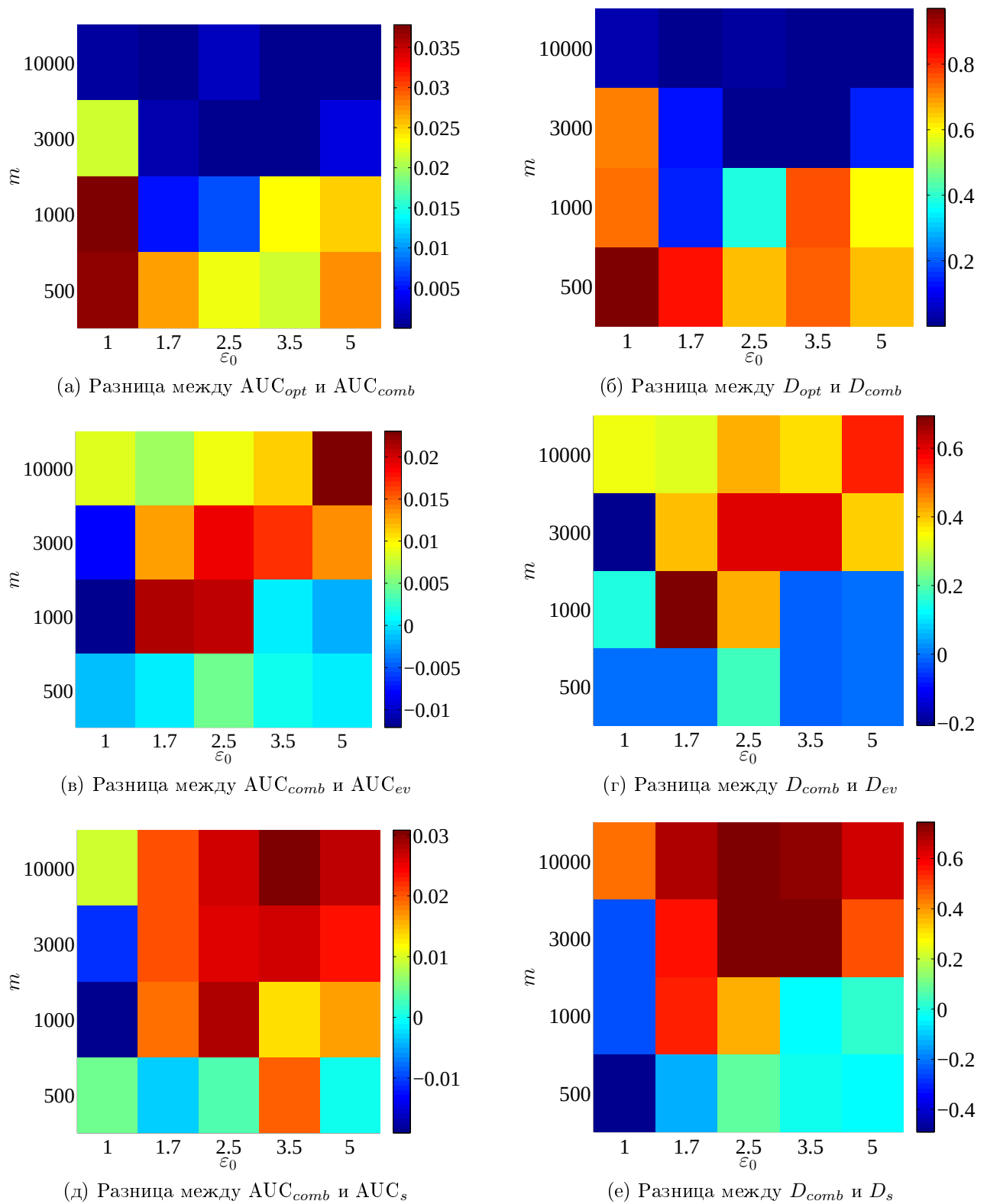
Рис. 5.19: Сравнение модели с комбинированными признаками с оптимальной моделью и моделью с исходными признаками для w_0 = 0.1
