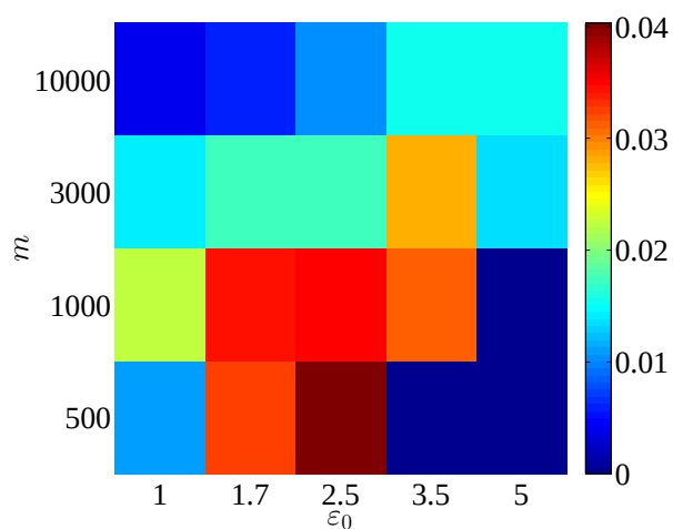
(в) Разница между AUC_{comb} и AUC_{ev}
