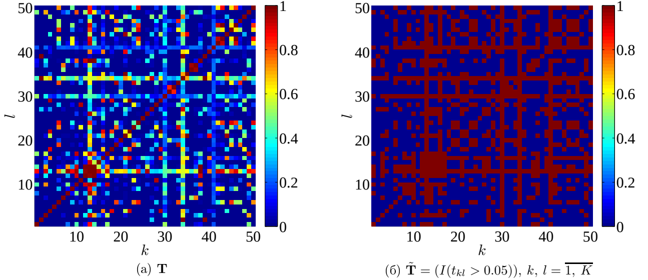
Рис. 5.12: Матрица парных уровней значимости в условиях истинности гипотезы о совпадении моделей
