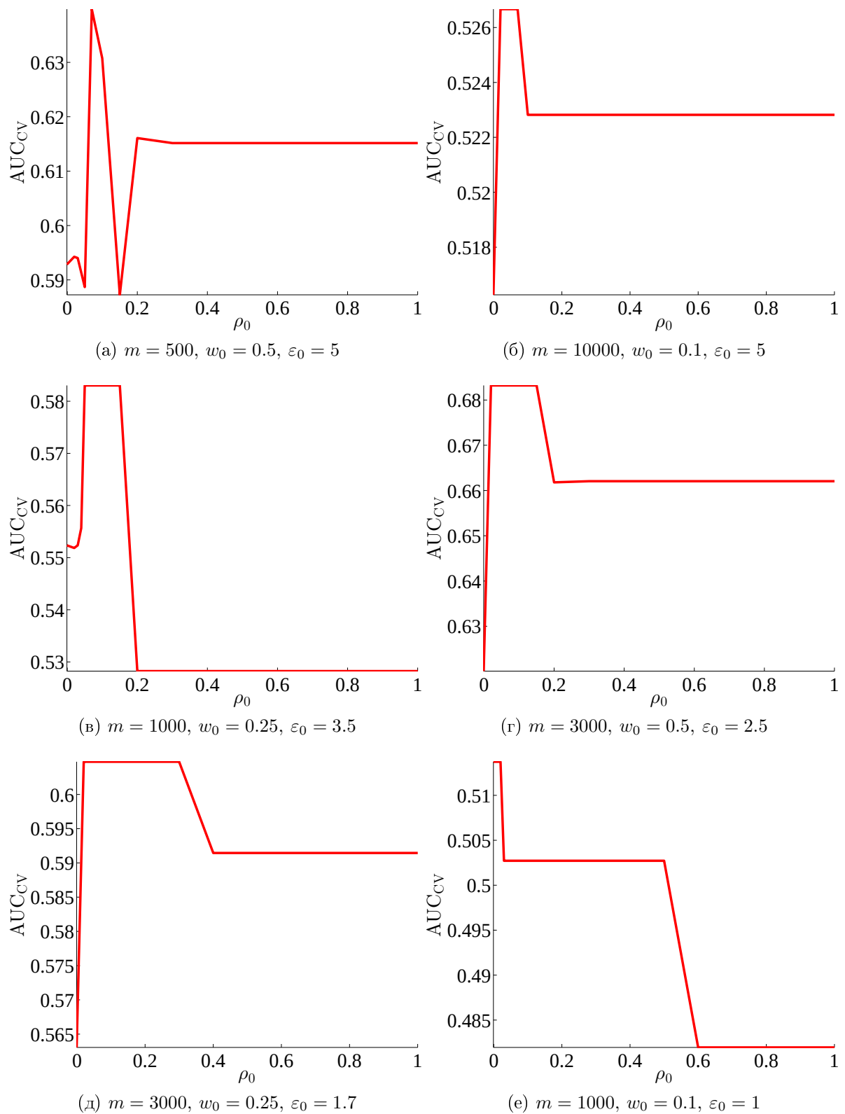
Рис. 5.18: Зависимость AUC на кросс-валидации от параметра отсечения по корреляции \rho_0 для разных m, w_0, \varepsilon_0 .
