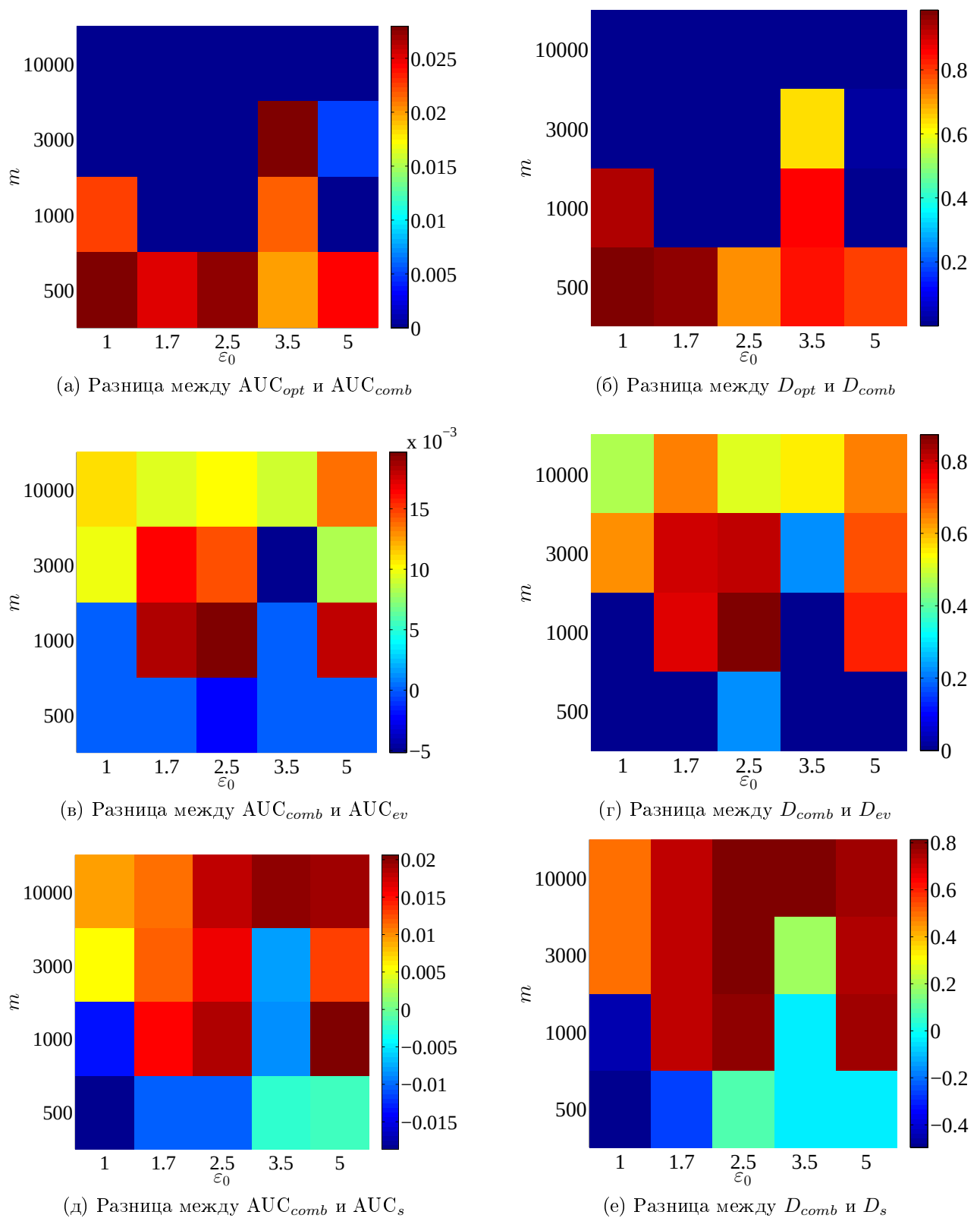
Рис. 5.15: Сравнение модели с комбинированными признаками с оптимальной моделью и моделью с исходными признаками для w_0 = 0.1
