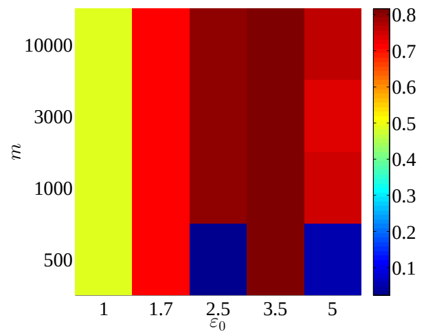
(е) Разница между D_{comb} и D_s
