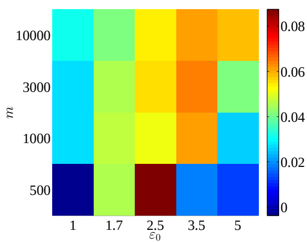
(д) Разница между AUC_{comb} и AUC_s
