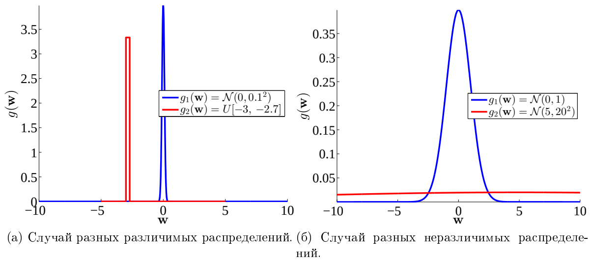
Рис. 4.1: Иллюстрация различий между отличием апостериорных распределений параметров пары моделей и различимостью моделей.
