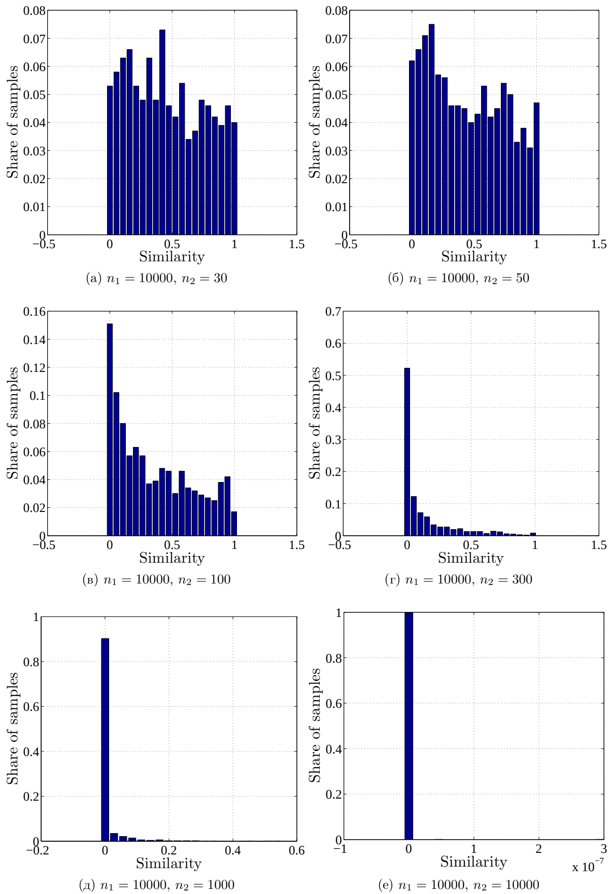
Рис. 5.1: Гистограмма распределения функции близости s-score s(g_1, g_2) для \rho = 0.95 в зависимости от числа объектов во второй выборке n_2
