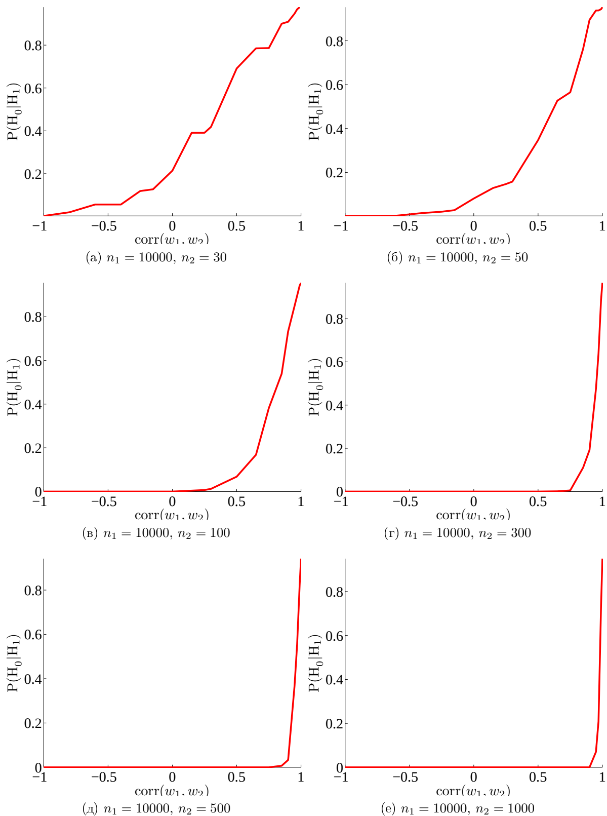
Рис. 5.4: Зависимость \mathbb{P}(H_0|H_1) от косинусной близости между истинными параметрами двух моделей \rho для разных значений числа объектов во второй выборке n_2
