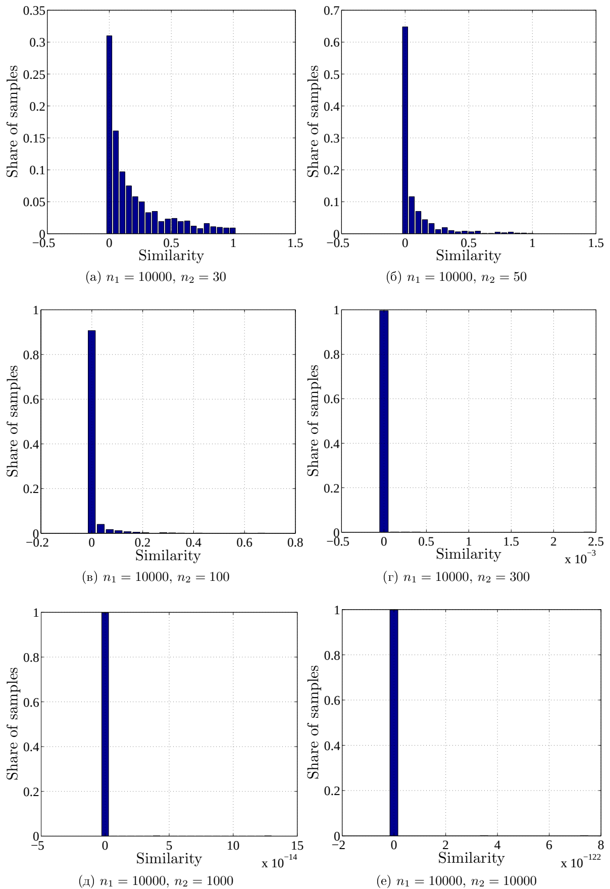
Рис. 5.3: Гистограмма распределения функции близости s-score s(g_1, g_2) для \rho = 0.5 в зависимости от числа объектов во второй выборке n_2
