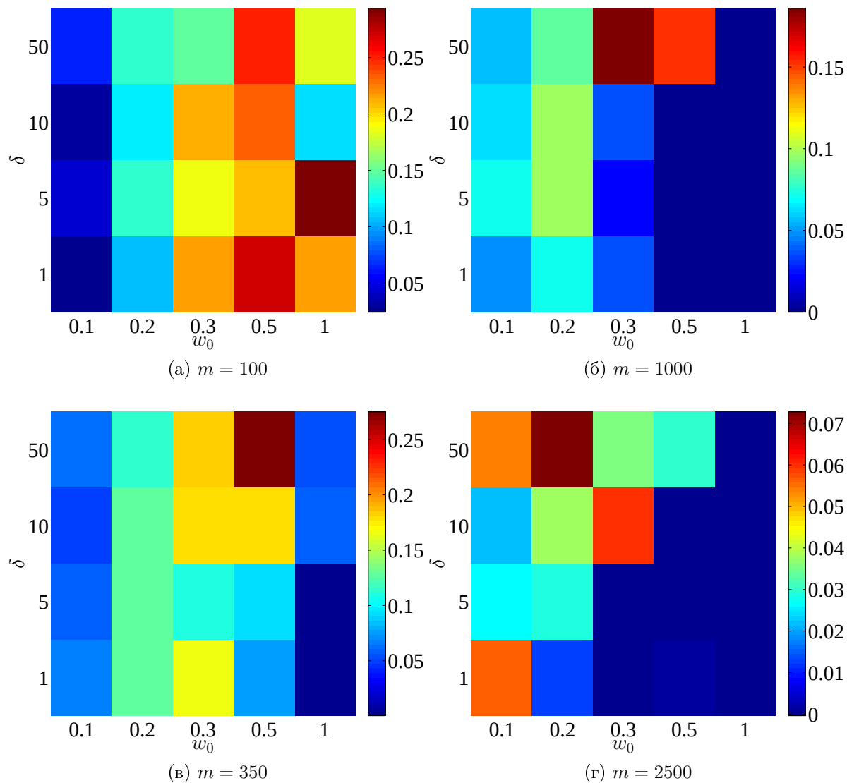
Рис. 5.9: Зависимость разности минимального AUC по кластерам для построенной (s, \alpha) – адекватной многоуровневой модели и исходной многоуровневой модели от m , \delta_0 и w_0 .
