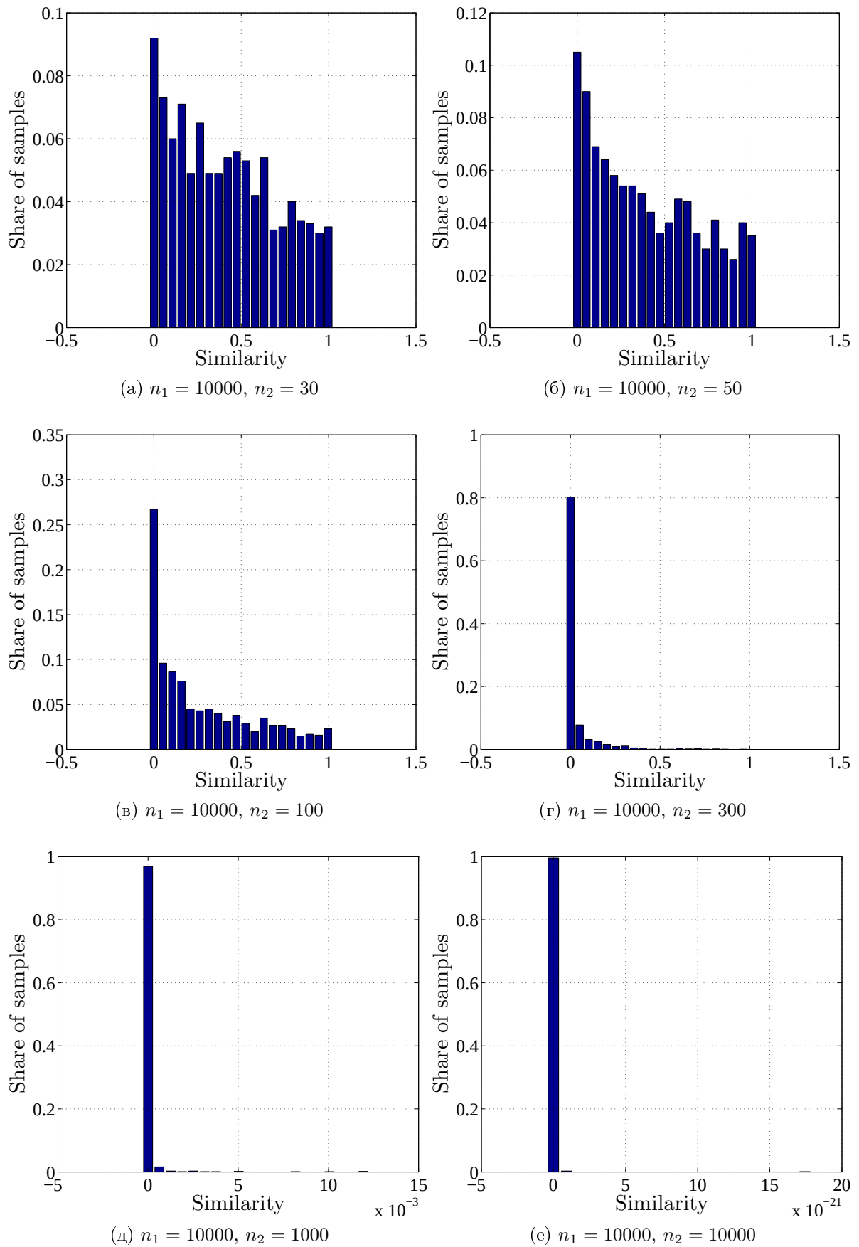
Рис. 5.2: Гистограмма распределения функции близости s-score s(g_1, g_2) для \rho = 0.9 в зависимости от числа объектов во второй выборке n_2
