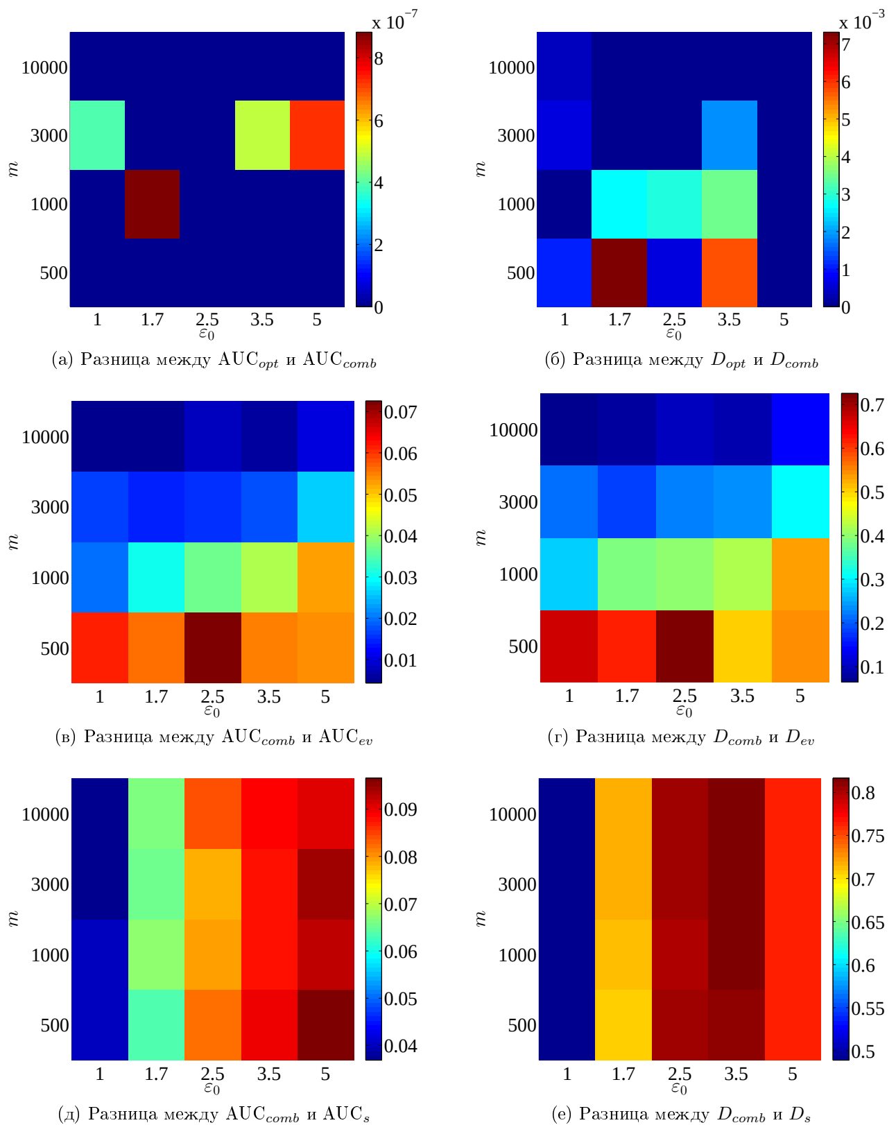
Рис. 5.17: Сравнение модели с комбинированными признаками с оптимальной моделью и моделью с исходными признаками для w_0 = 0.5
