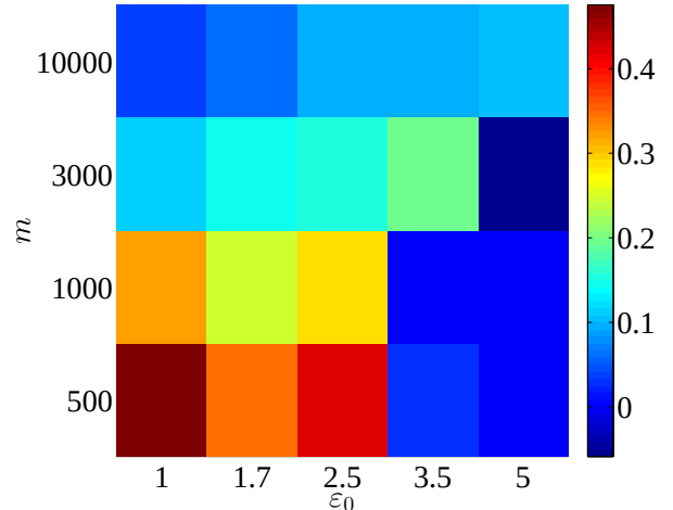
(г) Разница между D_{comb} и D_{ev}
