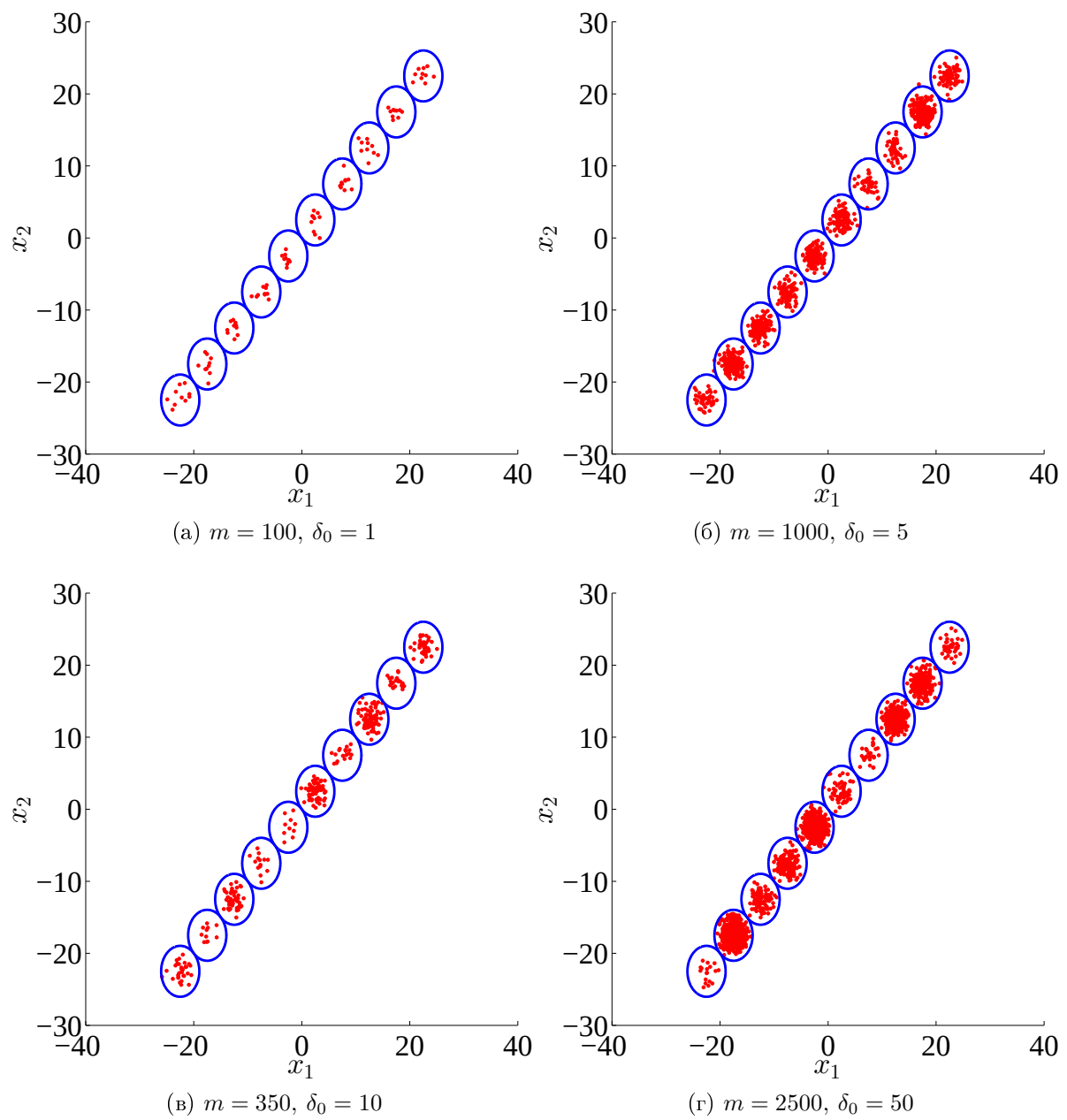
Рис. 5.5: Примеры сгенерированной синтетической выборки с кластерной структурой для разных значений m и \delta_0 .
