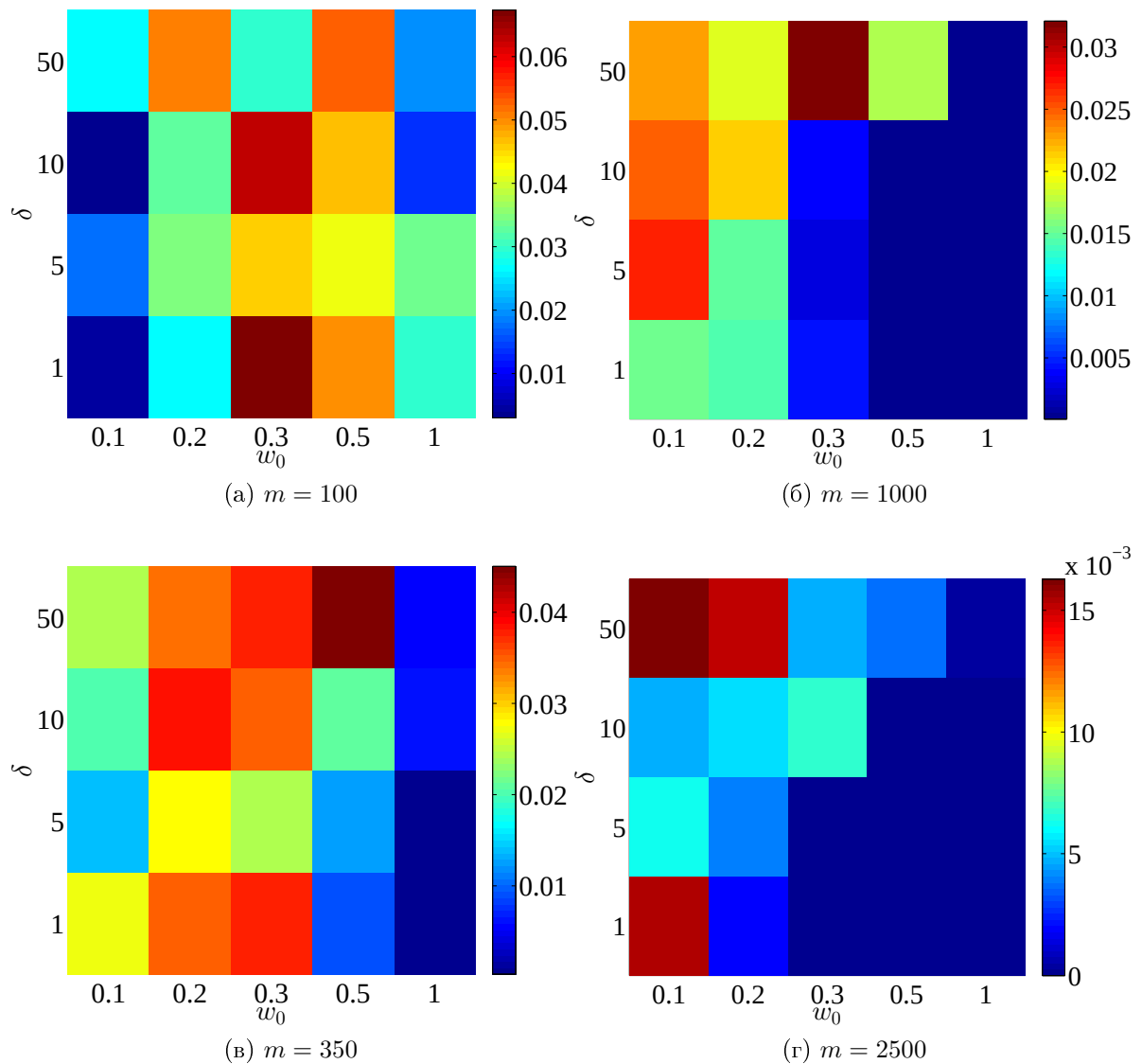
Рис. 5.8: Зависимость разности AUC для построенной (s, \alpha) – адекватной многоуровневой модели и исходной многоуровневой модели от m , \delta_0 и w_0 .
