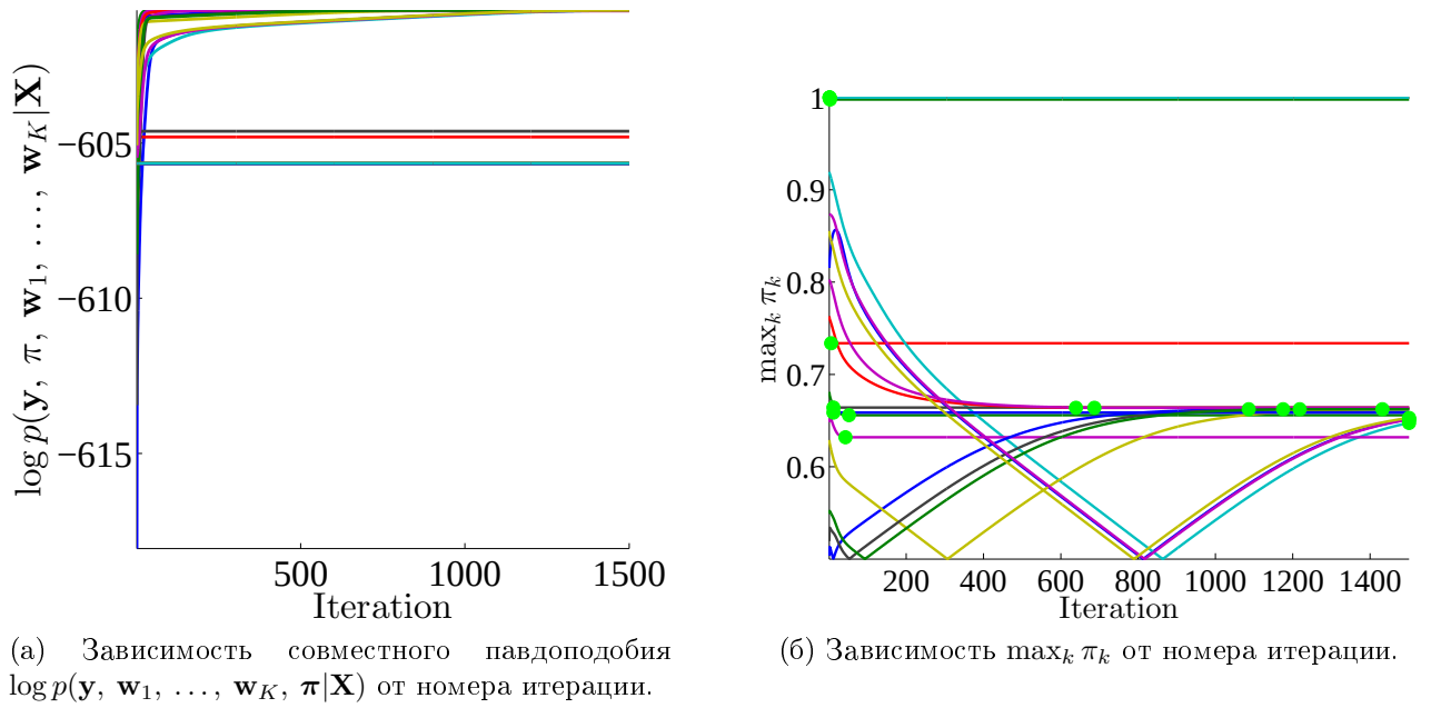
Рис. 5.11: Иллюстрация многоэкстремальности совместного правдоподобия смеси моделей.
