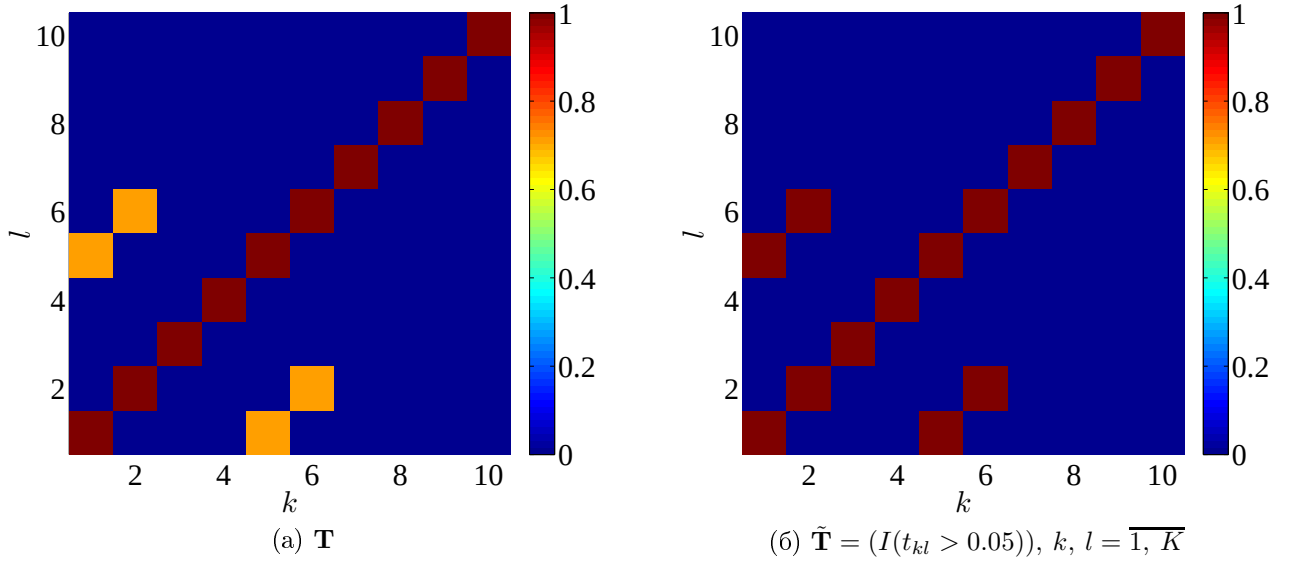
Рис. 5.13: Матрица парных уровней значимости в условиях истинности гипотезы о совпадении моделей
