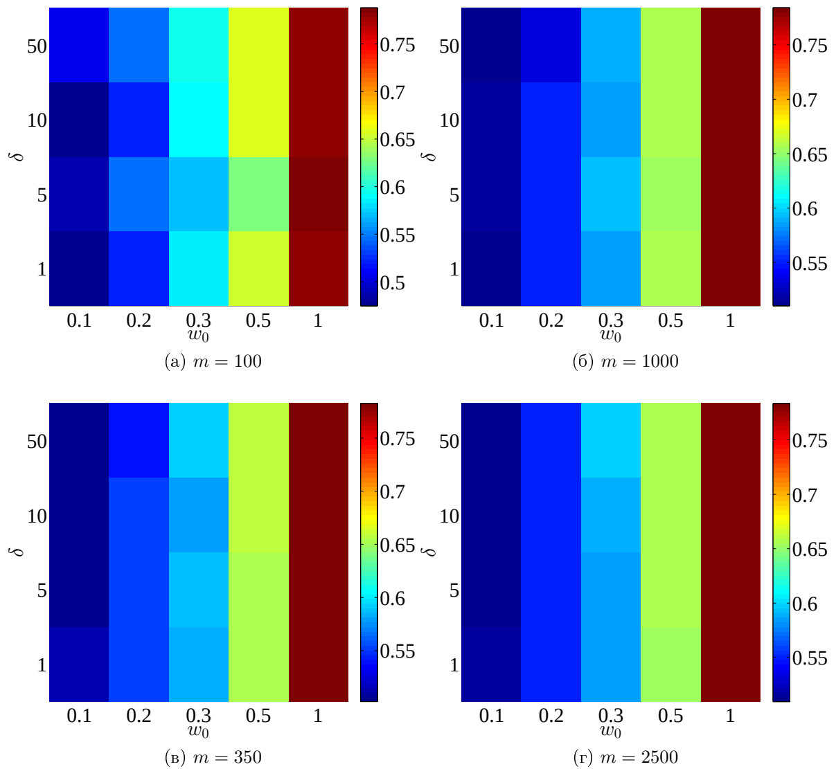
Рис. 5.7: Зависимость минимального AUC по кластерам от m , \delta_0 и w_0 для построенной (s, \alpha) – адекватной многоуровневой модели.
