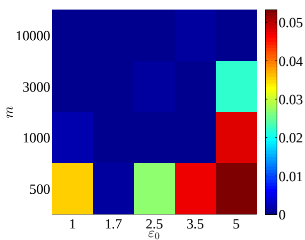
(а) Разница между AUC_{opt} и AUC_{comb}
