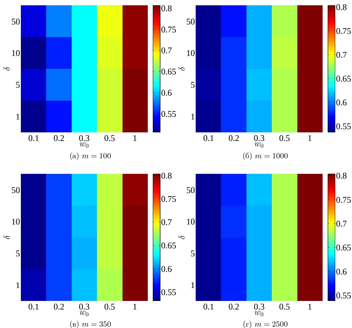
Рис. 5.6: Зависимость AUC от m , \delta_0 и w_0 для построенной (s, \alpha) – адекватной многоуровневой модели.
